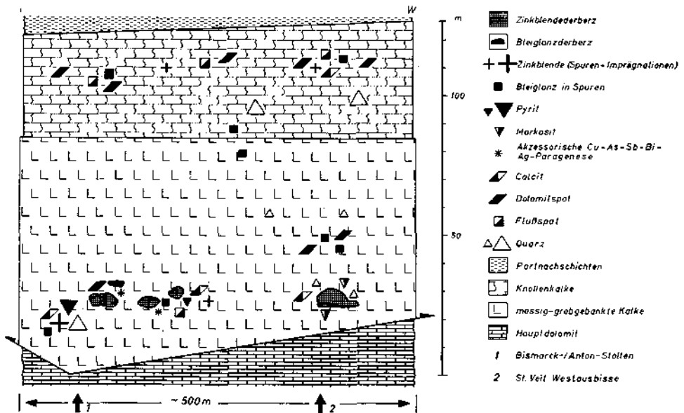
Abb. 3. Schematische Darstellung der stratigraphischen Position der Erzmineralparagenesen.
