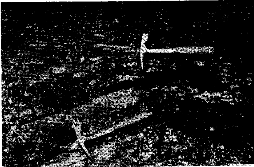
Abb. 1. Winkeldiskordanz zwischen oberdevonisch-unterkarbonischen Lyditen (untere Hälfte) und Sandsteinen und Schiefnern der Unteren kalkarmen Schichtgruppe (Auernigsschichten) am Weg zwischen Zollner Hütte und Colendiaul.
