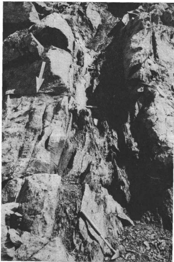
Abb. 3: Mylonitzone und steile Falte (Pfeil = Faltenachsenrichtung) am Scheibler
