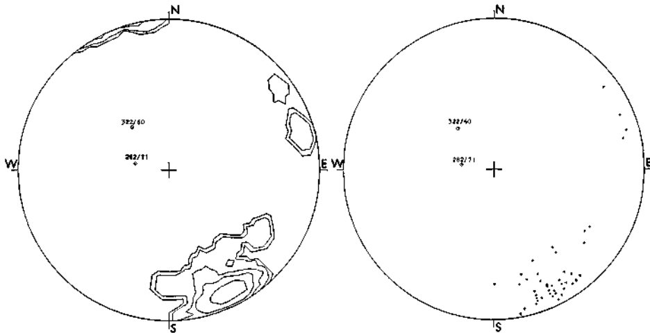
Abb. 8: Diagramme Küchelspitze; D 4 (links) aus Abb. 5. Polpunktediagramm (rechts)
