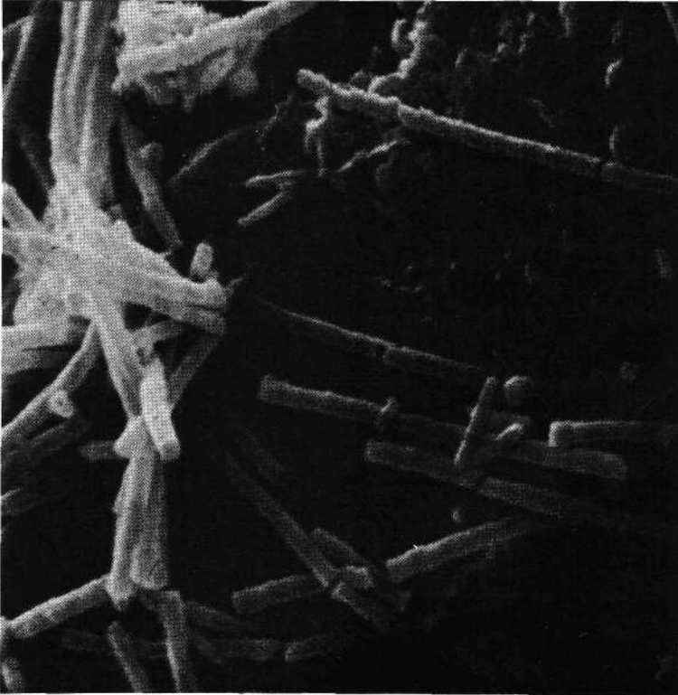
Abb. 6: Elektronenmikroskopische Aufnahme von Bleiglanzkriställchen im Halloysit.
