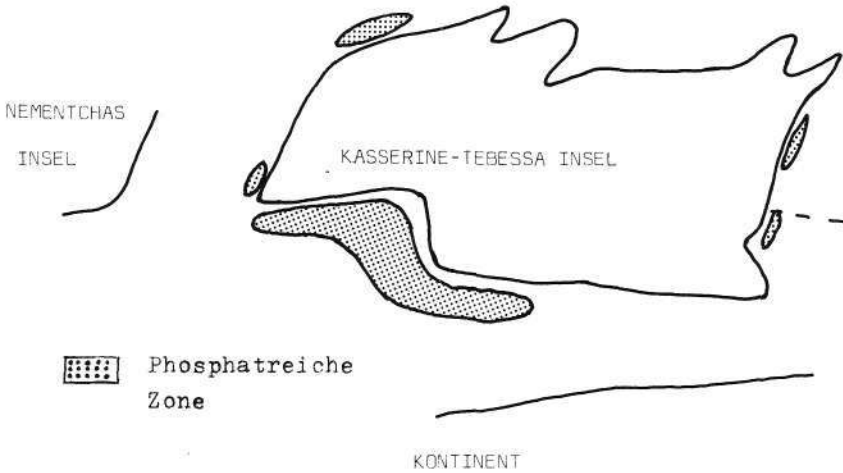
Abb. 2: Paleogeographische Verteilung der Phosphatlagerstätten des Mittleren Eozän.
