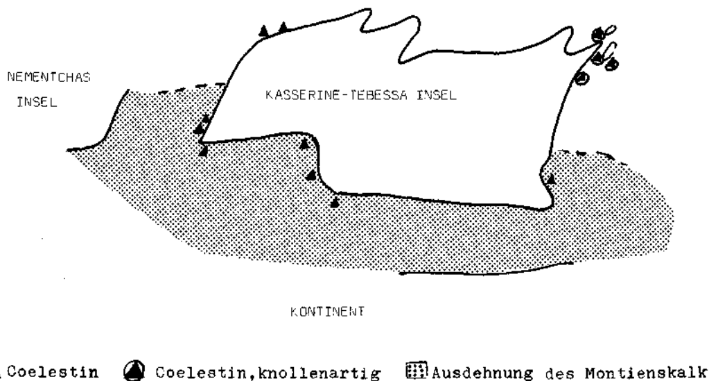
Abb. 1: Paleogeographische Verteilung der Coelestin-Vorkommen in Süd-Tunesien.
