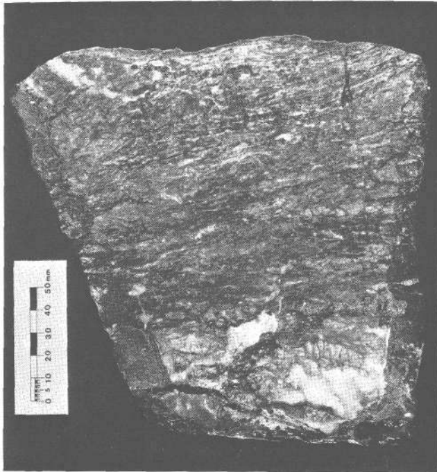
Abb. 5: Dörflerbachgraben bei Vorau (Oststeiermark). Detail aus konkordanter Lage von sideritischem Karbonat in „s“ (etwa waagrecht verlaufend) mit z. T. reichlich aufgesproßtem Granat (zumeist schwarz; stellenweise sind Kristalle erkennbar, z. B. an der Hangend- und liegendgrenze, am Kontakt zum Nebengestein, einem Granatglimmerschiefer). Gering mächtige Lagen von Granatglimmerschiefer (schwarz) treten vereinzelt auch im sideritischen Karbonat auf.
