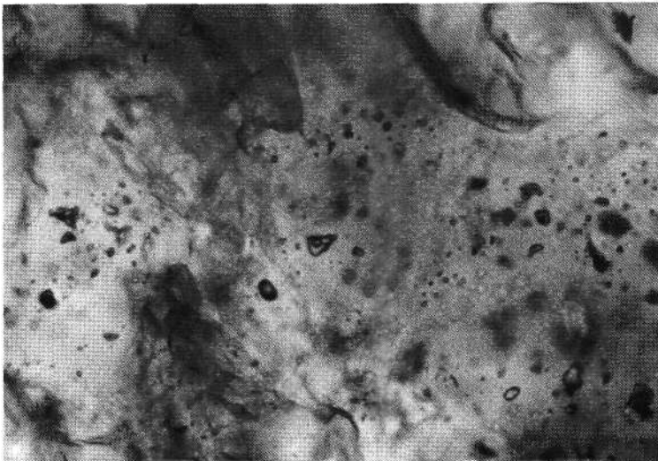
Abb. 22: Arzwaldgraben, Waldstein (Steiermark). Ausschnitt aus Baryt mit isoliertem zweiphasigen Flüssigkeits-Einschuß (Lösung und Gasblase – Bildmitte), der gesäumt wird von überwiegend einphasigen Einschlüssen. Polierter Dickschliff, Vergr.: 470 ×.
