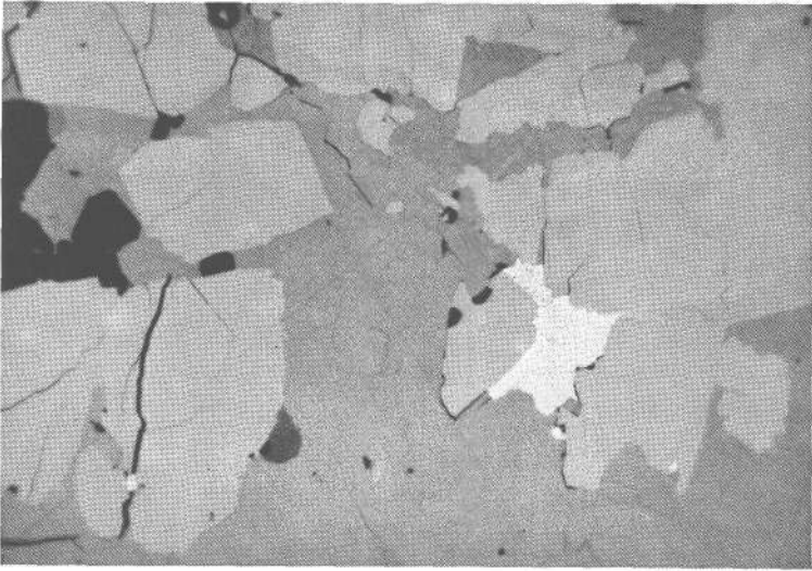
Abb. 13: Dörflerbachgraben bei Vorau (Oststeiermark). Gediegen Gold (Elektrum; fast weiß) in Verwachsung mit Kupferkies (mittelgrau; Hochtemperatur-Kupferkies) und teilweise idiomorph ausgebildetem Arsenkies (lichtmittelgrau in etwas unterschiedlichen Tönen – Reflexionspleochroismus). Daneben tritt etwas Magnetkies (dunkelgrau) und Gangart (schwarz) auf. Anschliff, Ölimmersion, Vergr.: 375×.
