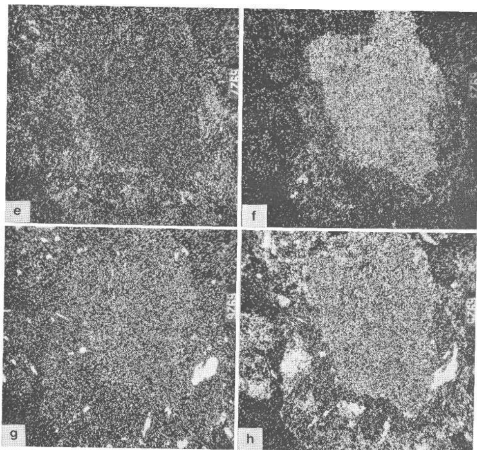
Abb. 3b: Profil Stob 1, Probe 1; Titanit mit deutlich abgrenzbarer Verwitterungsrinde. e)–h) Verteilungsbilder von K, Ca, Ti, Fe
