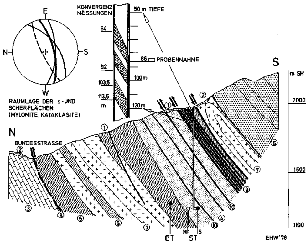
Abb. 1: Querschnitt durch den Albona-Schacht (W-Bereich des Arlbergstraßentunnels). 1 = Moorbildungen; 2 = Gehängeschutt, Moräne; 3 = Permtrias der nördlichen Kalkalpen; 4 = Feldspat-knotengneiss; 5 = Biotitplagioklasgneiss; 6 = Gneissphyllite (Schiefergneiss bis Glimmerschiefer, Phyllite, Phyllonite); 7 = Muskovitgranitgneiss; 8 = Tektonische Naht (Kalkalpen-Kristallin); 9 = Aufschiebungstektonik der Silvrettadecke: Bewegungsbahnen mit vornehmlich mächtigen Myloniten im s-Gefüge; 10 = Scherflächen mit Myloniten; ST = Straßentunnel; S = Röhre Süd; N = Röhre Nord; ET = Eisenbahntunnel
