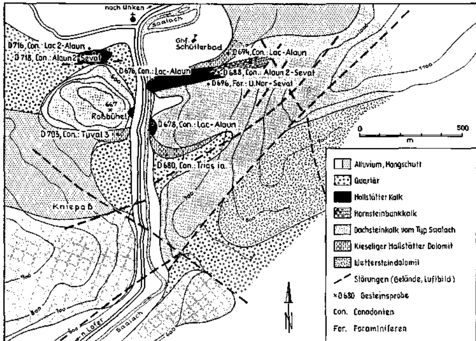
Abb. 1: Geologische Karte und Beprobungsplan der Hallstätter Kalkvorkommen im Bereich der Saalach-Stirnschuppe (Berchtesgadener Decke) südlich Unken
