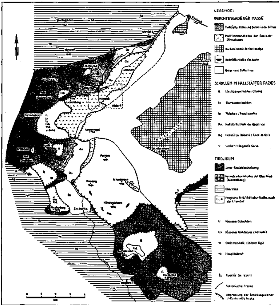
Abb. 4: Die Faziesverhältnisse am Westrand der Berchtesgadener Masse
