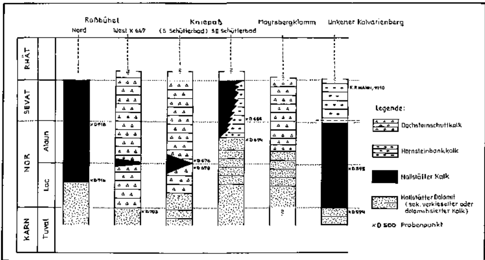
Abb. 2: Profile der Faziesverzahnungen von Hallstätter- und Dachsteinkalkfazies im Bereich der Saalach-Stirnschuppe (Berchtesgadener Decke) südlich Unken
