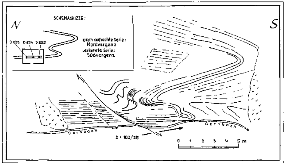
Abb. 8: Großräumig verfaltete Jura-Neokomkalke, Fußweg Gernbach, 300 m südlich Kirche Vordergern, SE Gschirrkopf, nördlich Berchtesgaden
