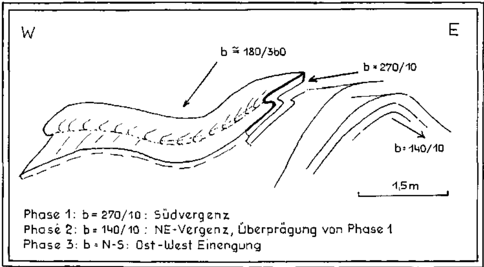
Abb. 7: Potenzierte Faltung in den Jura/Kreideschichten der Unkener Mulde, Weg NW Kapelle 847 Hintergföll, 5,52 km westlich Unken
