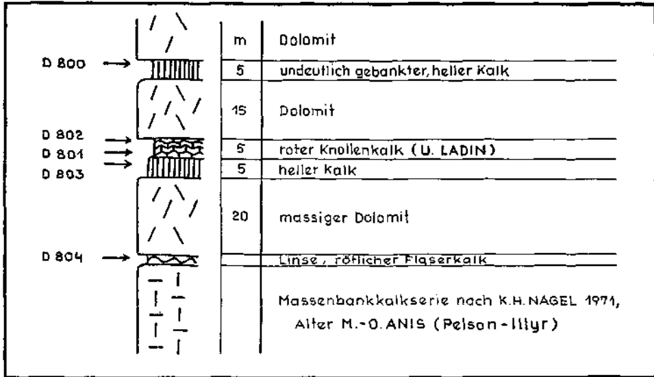
Abb. 3: Profil Kienberg Süd. Einschaltung von ladinischen Hallstätter Kalken innerhalb der dolomitisierten Mitteltrias am Südwestrand der Berchtesgadener Masse (vgl. Abb. 4)
