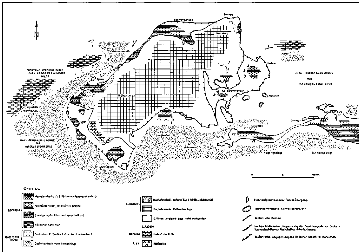
Abb. 5: Schematische Faziesgliederung der westlichen Hallstätter Zone (Obertrias und lokal Mitteltrias). Tektonofazielle Abgrenzung nach F. F. HAHN (1910 Fig. 14 und 15) sowie A. TOLLMANN (1976c, Karte), verändert umgezeichnet
