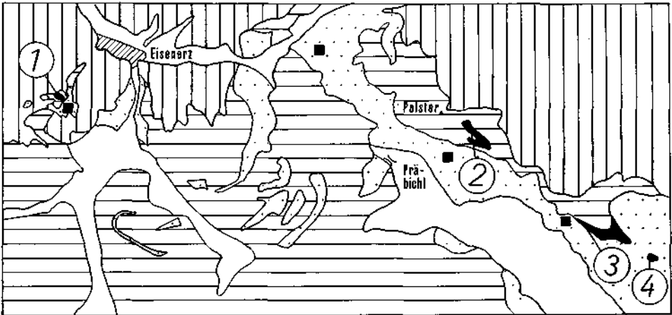
■ Polster Quarzit ▨ Blasseneck Porphyroid ▤ Paläozoikum der Grauwackenzone ▧ Nördliche Kalkalpen □ Quartär
