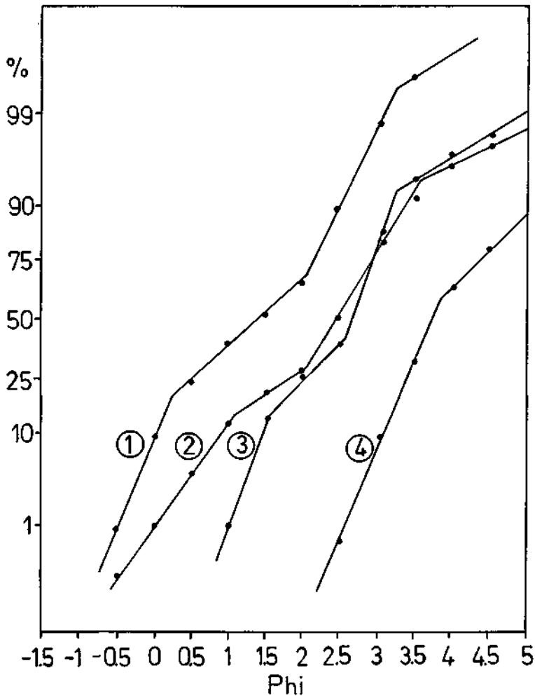
Abb. 4: Korngrößensummenkurven im Wahrscheinlichkeitsnetz: 1 = basale Quarzarenite, 2 = Kalksandsteine, 3 = Quarzwackenbasis, 4 = feinkörnige Quarzwacken
