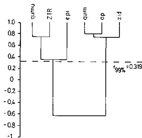
Abb. 6: Cluster-Diagramm von sechs Variablen (Abkürzungen s. Tab. 6) mit dem Produkt-Moment-Korrelationskoeffizienten ( r ) als Ähnlichkeitsmaß
