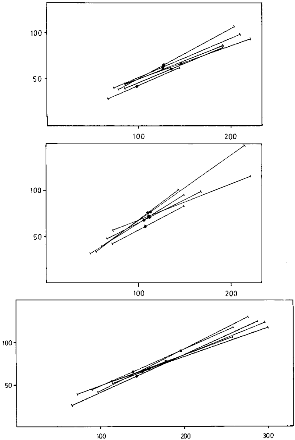
Abb. 3: RMA-Diagramme: a) idiomorpher Zirkon, Polster-Quarzit, b) gerundeter Zirkon, Polster-Quarzit, c) idiomorpher Zirkon, Blasseneck-Porphyr. Mittlere Zirkonlängen und -breiten sind durch ● gekennzeichnet
