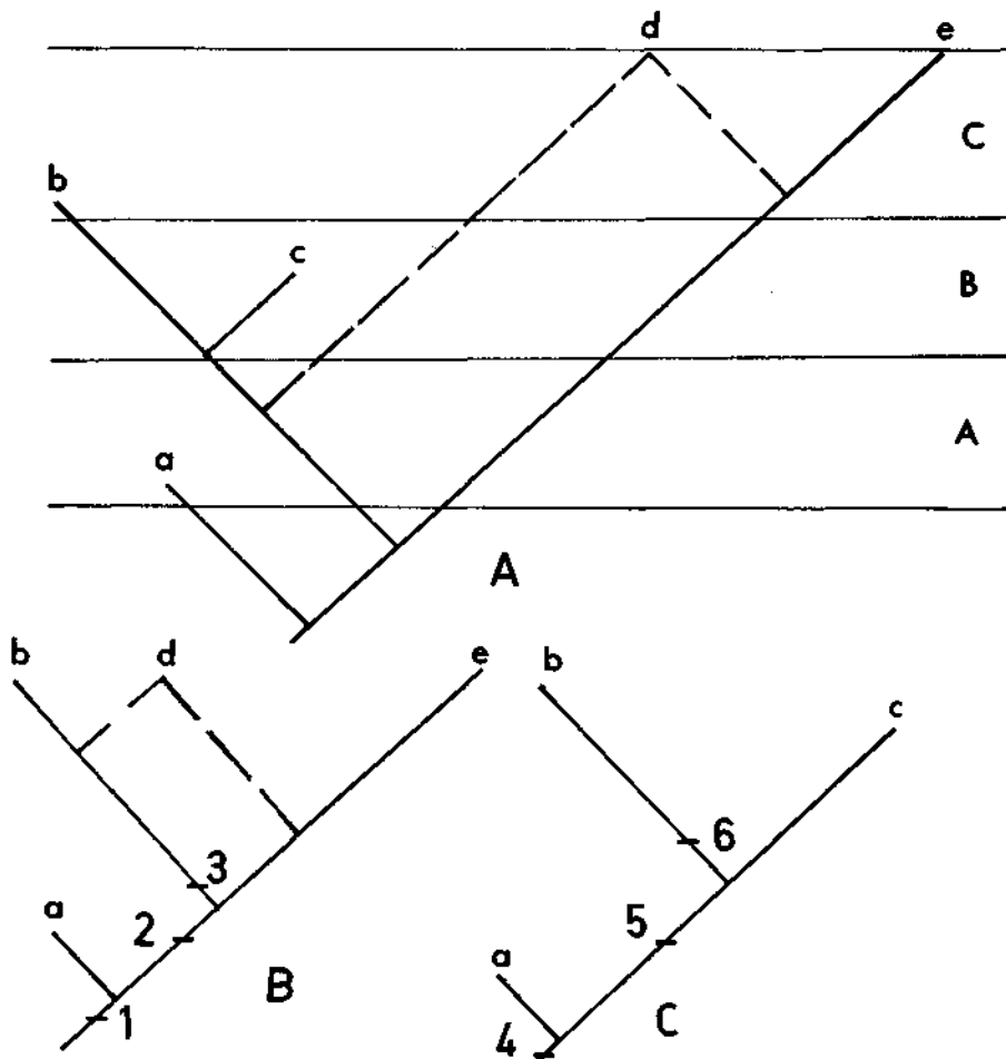
Abb. 4: Verwandtschaftsbeziehungen Triassischer Dipnoer der Gruppe von Tellerodus sturii ; A nach allen Merkmalen, B nach den Zahnplatten, C nach den Schädeldächern. A: Untertrias, B: Mitteltrias, C: Obertrias.
