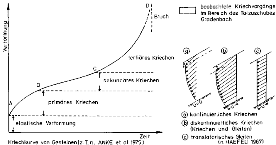
Abb. 5: Kennzeichnung von Kriechvorgängen mit Hilfe der Verformung, der Zeit und des Raumes und ihre mögliche Zuordnung im Bereich des Talzschubes Gradenbach.
