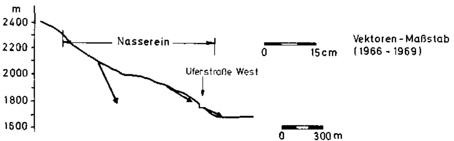
Längsprofil Sackung Nasserein - Gepatschspeicher/Kaunerital (n. NEUHAUSER u. SCHÖBER 1970)
