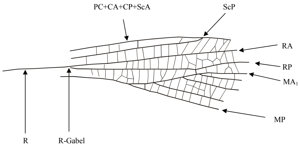
Abb. 5: Zeichnerische Rekonstruktion des rechten Mesothorakflügels (Vorderflügels) von Hirsutgerarus saxonicus n. gen. n. sp.
