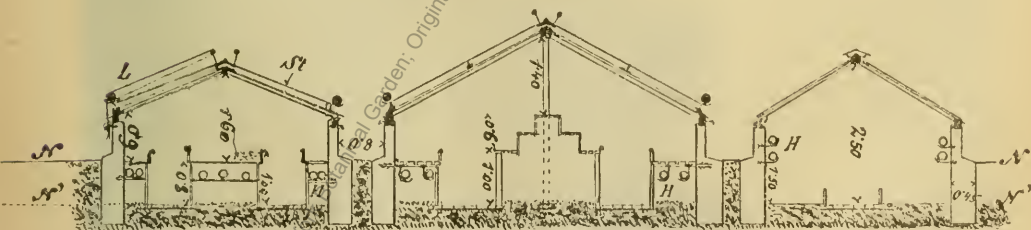
Fig. 51. Glashäuser im Culturgarten zu Ferrières-en-Brie. (Nach rechts schliessen sich mehrere Häuser derselben Art an.)
