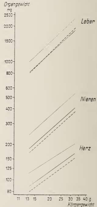
Abb. 2. Beziehungen zwischen dem Gewicht von Herz, Leber und Nieren und dem Nettokörpergewicht bei weiblichen Albinomäusen, die 40 h geschwommen hatten (— — — —), bei unter Laborbedingungen gehaltenen weiblichen Albinomäusen (— — — —) und bei weiblichen Waldmäusen (.....). Nach CLASS, Z. Anat. 122, 260. 1961
