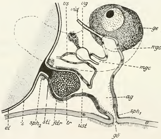
Fig. 1. Polycystis goettei . Geschlechtsorgane in Seitenansicht. Etwa 230 \times . ag, Atrium genitale; ei, Eikapsel; fdr, Filamentdrüsen; ge, Germarium; gö, Geschlechtsöffnung; mge, männl. Genitalkanal; sph 1 u. sph 2 , Sphinctere; sti, Stielchen; tr, Filamenttropfen; u, Uterus; ust, Uterusstiel; vg, Vesicula granulorum; vi, Vitellarien; vid, Vitelloduct; vs, Vesicula seminalis; rge, weibl. Genitalkanal (Ductus communis).
