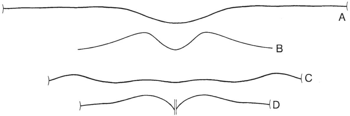
Abb. 53: Verlauf der Anwachsstreifen und Einschnürungen bei Acutimitoceras aus dem Hangenberg-Kalk des Bahneinschnittes von Ober-Rödinghausen (A-C, coll. VÖHRINGER) und Bank 21 von Gattendorf (D, coll. SCHINDEWOLF).
