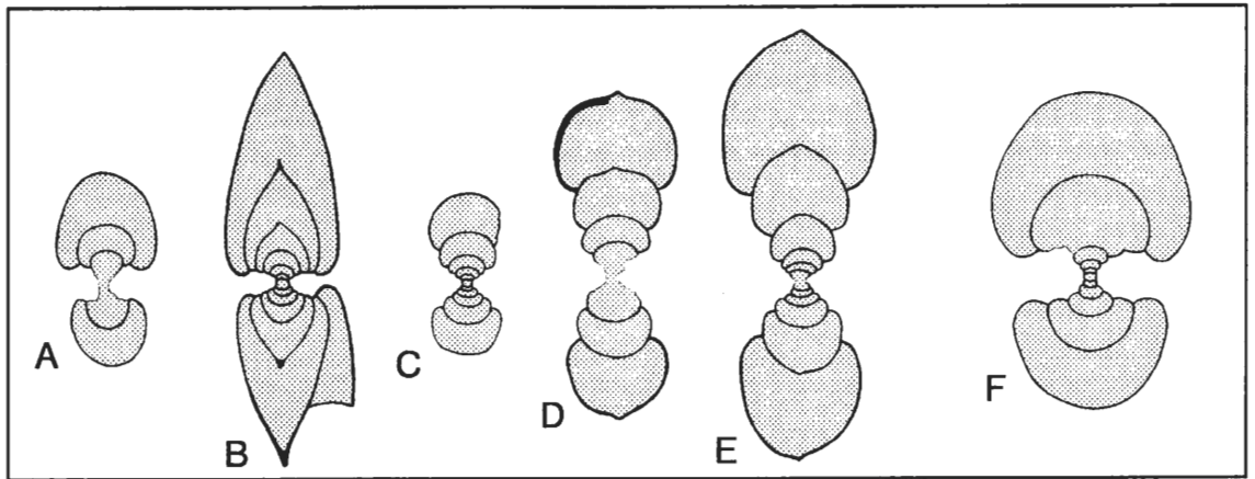
Abb. 71: Querschnitte verschiedener Goniatiten aus dem Hangenberg-Kalk des Bahneinschnittes von Ober-Rödinghausen (A-E, coll. VÖHRINGER) und der prorsum -Zone vom Müszenberg (coll. KORN 1978), x 2,5.
