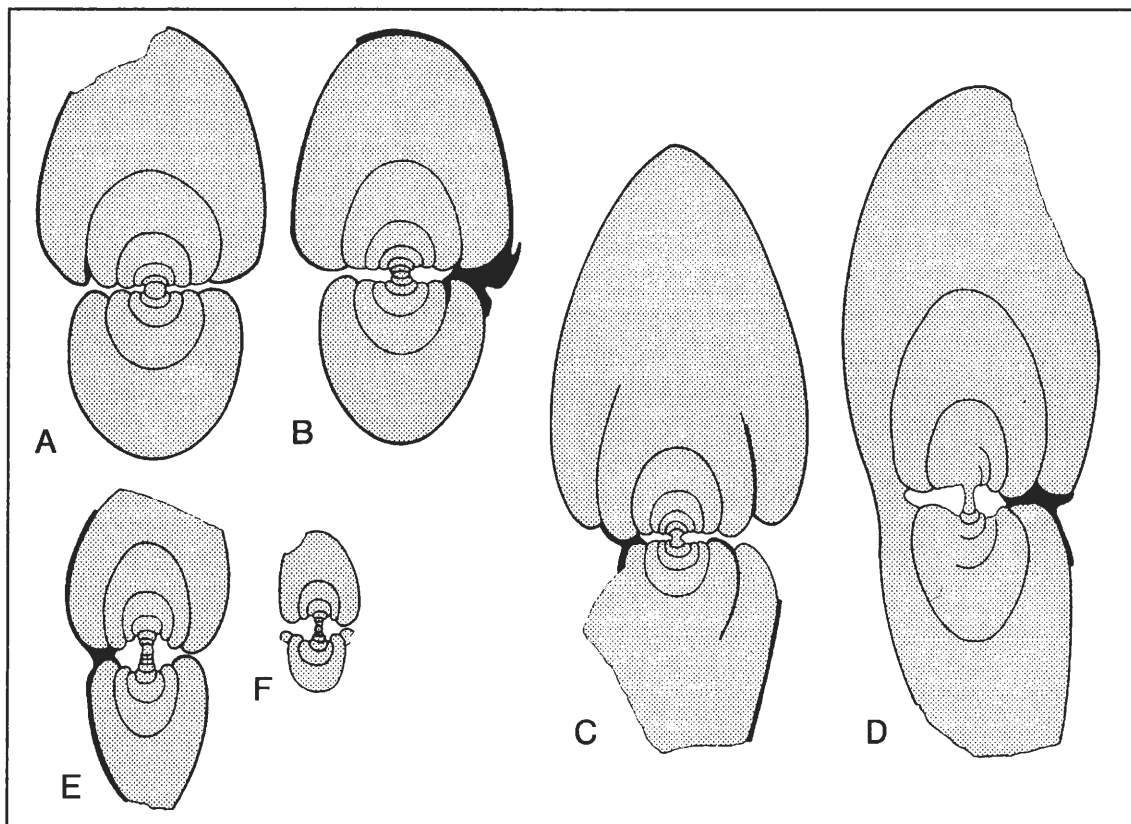
Abb. 59: Querschnitte von Nicimitoceras aus dem Hangenberg-Kalk des Bahneinschnittes von Ober-Rödinghausen, x 2,5. Alle Exemplare coll. VÖHRINGER.
