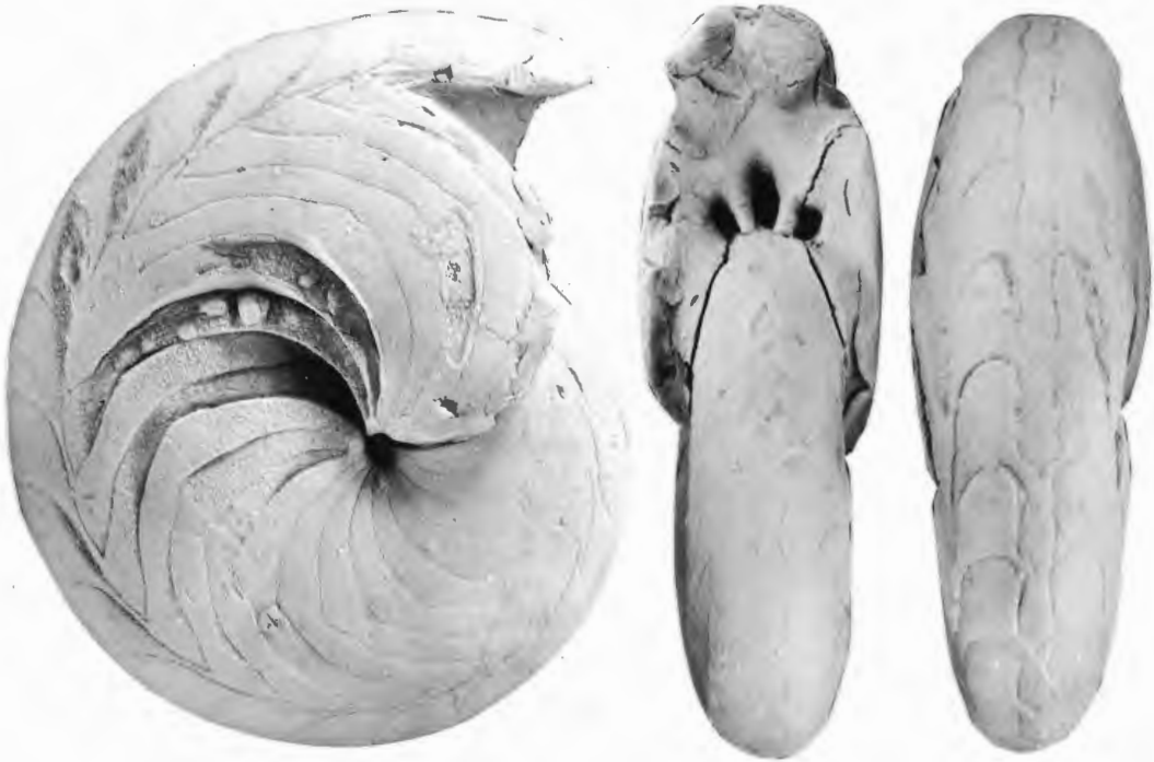
Abb. 34: Imitoceras ixion (HALL 1860) aus dem Rockford Limestone von Rockford, Indiana; GPIT 1748/1; x 1.
