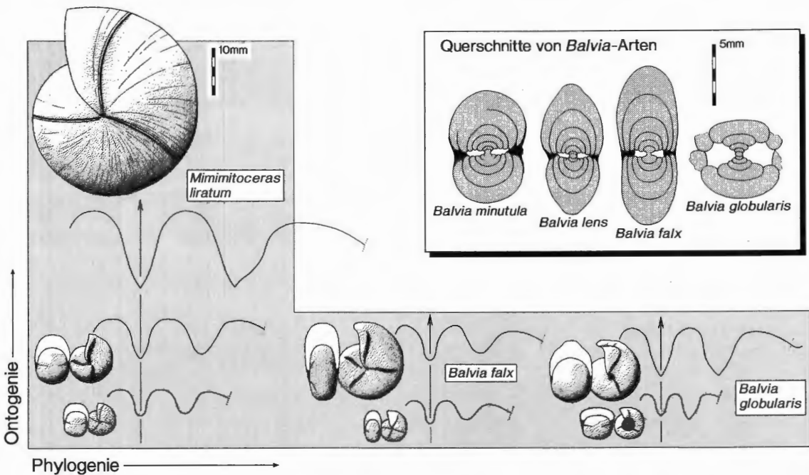
Abb.3: Das Verhältnis von Ontogenie und Phylogenie in der Evolution von Mimimitoceras und Balvia (aus KORN 1992).
