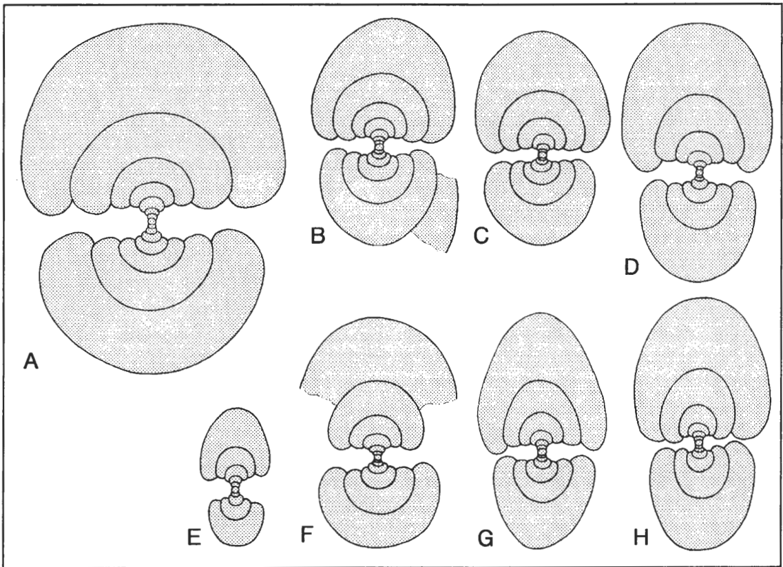
Abb. 37: Querschnitte von Acutimitoceras und Nicimitoceras aus dem Stockumer Kalk von 900m ESE Stockum, x 2,5. Alle Exemplare coll. KORN 1982.
