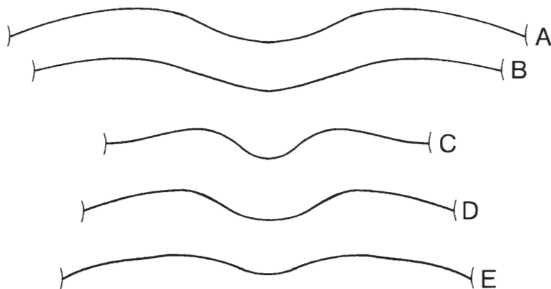
Abb. 54: Verlauf der Anwachsstreifen und Einschnürungen bei Acutimitoceras aus dem Hangenberg-Kalk des Bahneinschnittes von Ober-Rödinghausen. Alle Exemplare coll. VÖHRINGER.
