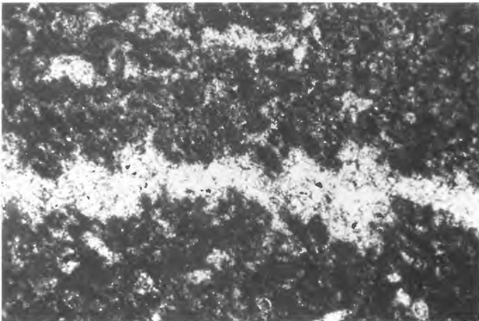
Abb. 3: Planare LF-A-Gefüge; Steinbruch Frettholz. Dünnschliff, Vergr. 30x.
