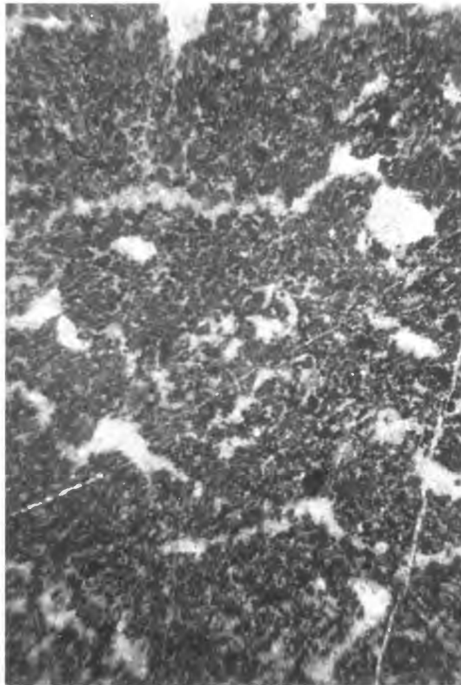
Abb. 4: Unregelmäßige LF-A-Gefüge; Steinbruch Frettholz. Dünnschliff, Vergr. 8x.
