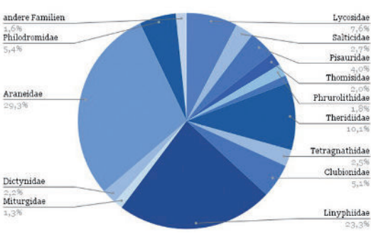
Kreisdiagramm zur prozentualen Verteilung der Spinnenfamilien während der gesamten Messungen (2085 Individuen)
