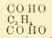
Bernsteinsäure,
