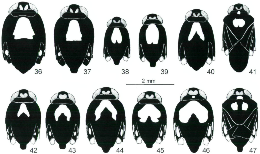
Abb. 36 - 47: Schematische Darstellungen der Körperformen und Farbmuster bei philippinischen Arten der Gattung Esakia ; Körperanhänge bis auf Meso- und Metacoxa sowie Behaarungen und die meisten Suturen weggelassen: (36, 37) E. usingeri (nach Material aus Luzon, Isabela Prov., in Coll. V.P. Gapud, Los Baños), (38 - 41) E. palawanensis sp.n., (42 - 47) E. cenizae sp.n. (42 - 44, 47: aus Samar, 45, 46: aus Bohol); (36, 40, 44) ungeflügeltes Weibchen; (37 - 39, 42, 43, 45) ungeflügeltes Männchen; (41) geflügeltes Männchen; (47) geflügeltes Weibchen mit selbstmutilierten Flügeln.
