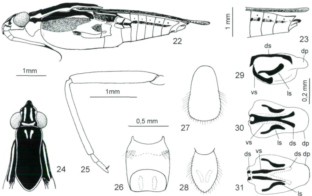
Abb. 22 - 31: Limnogonus anderseni sp.n., Behaarungen ganz oder teilweise weggelassen: (22) Habitus des makropteren Männchens, lateral; (23) Abdomenende des makropteren Weibchens, lateral; (24) Kopf und vorderer Thoraxbereich des apteren Männchens, dorsal; (25) Vorderbein des apteren Männchens; (26) Segment 8 ( \sigma ); (27) Pygophor ( \sigma ); (28) Proctiger ( \sigma ); (29 - 31) Vesicula-Sklerite: (29) lateral, (30) dorsal, (31) ventral; dp - Dorsalplatte, ds - Dorsalsklerit, ls - Lateralsklerit, vs - Ventralsklerit.
