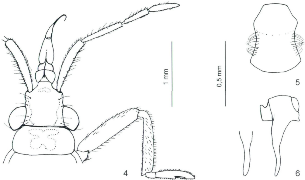
Abb. 4 - 6: Stenobatopsis coronensis sp.n., Männchen: (4) Kopf mit Antenne und Rostrum (nach vorne geschlagen), Pronotum und Vorderbein, dorsal; (5) Pygophor, ventral; (6) Proctiger, lateral, und Proctiger-Fortsatz in Frontalansicht; Behaarungen teilweise weggelassen.
