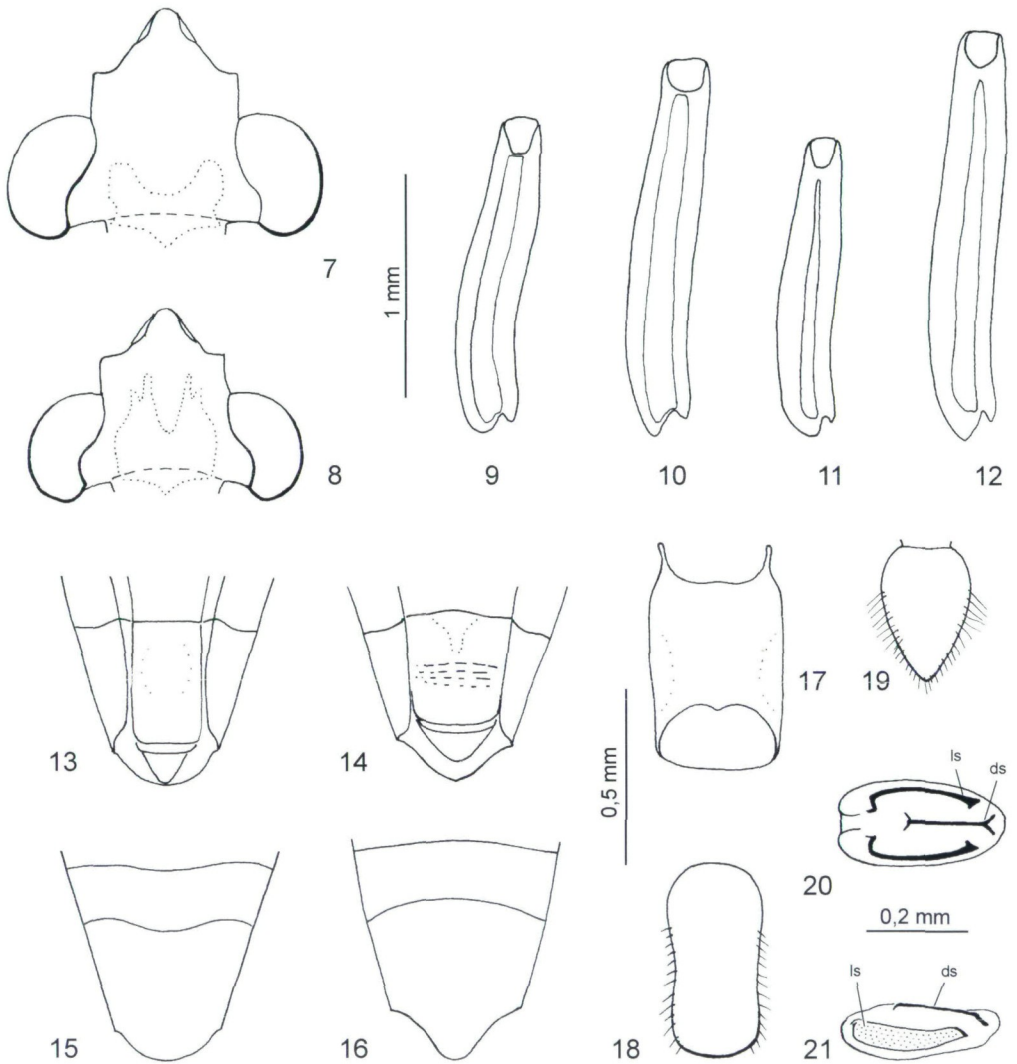
Abb. 7 - 21: (7, 9, 10, 13, 15, 17 - 21) Neogerris philippinensis sp.n.; (8, 11, 12, 14, 16) Neogerris parvulus : (7, 8) Kopf, dorsal; (9 - 12) Femur, Beugeseite, Umrandung zeigt Ausdehnung der schwarz beborsteten Fläche (9, 11: Männchen; 10, 12: Weibchen); (13, 14) Abdomenende des apteren Weibchens, dorsal; (15, 16) 6. und 7. Sternit des Weibchens, ventral; (17 - 21) Genitalia des Männchens: (17) 8. Segment, ventral; (18) Pygophor, ventral; (19) Proctiger, dorsal; (20) Vesikulasklerite, dorsal; (21) Vesikulasklerite, lateral (ds - Dorsalsklerit; ls - Lateral-sklerit); Behaarungen ganz oder teilweise weggelassen.
