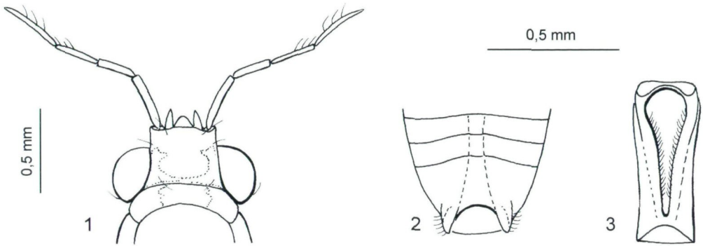
Abb. 1 - 3: Rhagadotarsus palawanensis sp.n., Holotypus, apteres Männchen: (1) Kopf und Pronotum, dorsal; (2) 5. - 7. Sternit, ventral; (3) 8. Segment, ventral.
