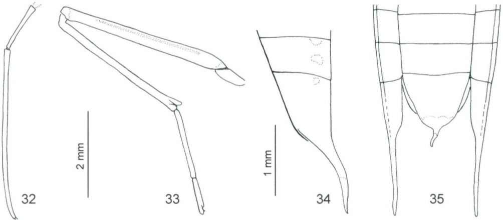
Abb. 32 - 35: Potamometropsis longipes sp.n., Holotypus, apteres Weibchen, Behaarung weggelassen: (32) 1. und 2. Antennenglied; (33) Vorderbein; (34) 6. und 7. Sternit, lateral; (35) Abdomenende, dorsal.
