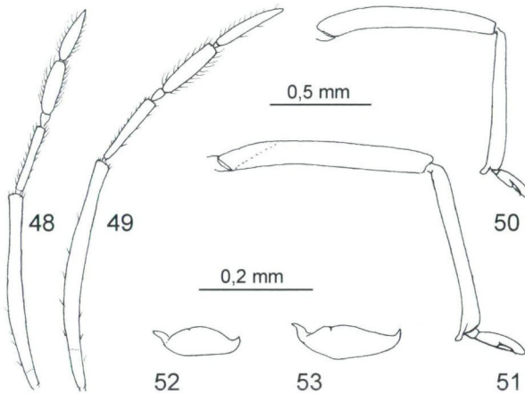
Abb. 48 - 53: (48, 50, 52) Esakia palawanensis sp.n., (49, 51, 53) Esakia cenizae sp.n.: (48, 49) Antenne des Männchens; (50, 51) Vorderbein des Männchens; (52, 53) linke Paramere, lateral; Behaarungen ganz oder teilweise weggelassen.
