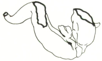
Fig. 3 a. Diceras bubalinum Peters. Skizze. Die Abplattungsebene ist in waagrechte Lage gebracht. — Die Orientierung im Sediment ist völlig verschieden von Fig. 1 a und 2 a. Auch die Wirbelspitze des Steinkernes ist ebenfalls abgeplattet. Originale befinden sich im Naturhistorischen Museum, Wien.
