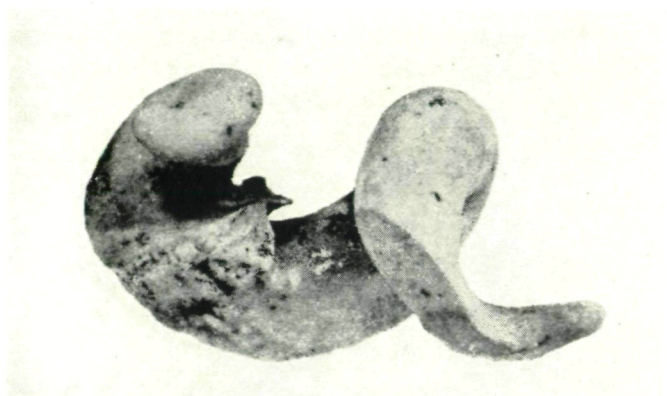
Fig. 1. Dicerus bubalinum Peters. Unvollkommener Steinkern. Ob. Jura Dörfles bei Ernstbrunn Steinbr. 1. Natürl. GröÙe.
