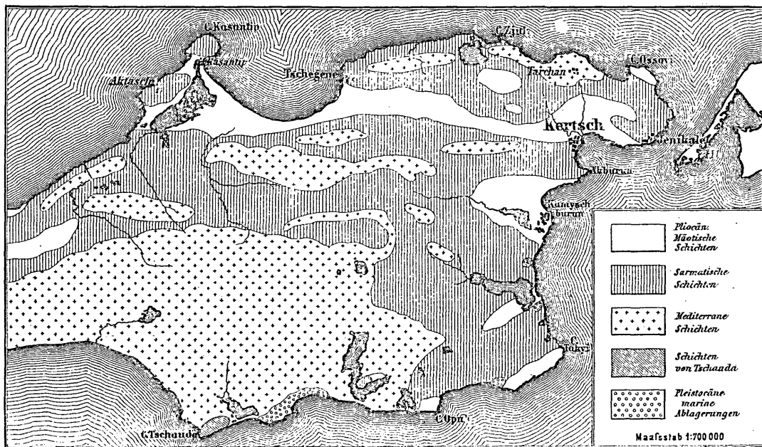
Geologische Skizzenkarte der Halbinsel Kertsch.
