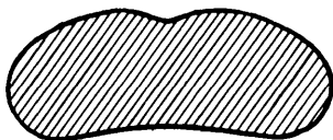
Abb. 4. Discoaster claviger nov. spec. Achsialschnitt. 4400\times .
