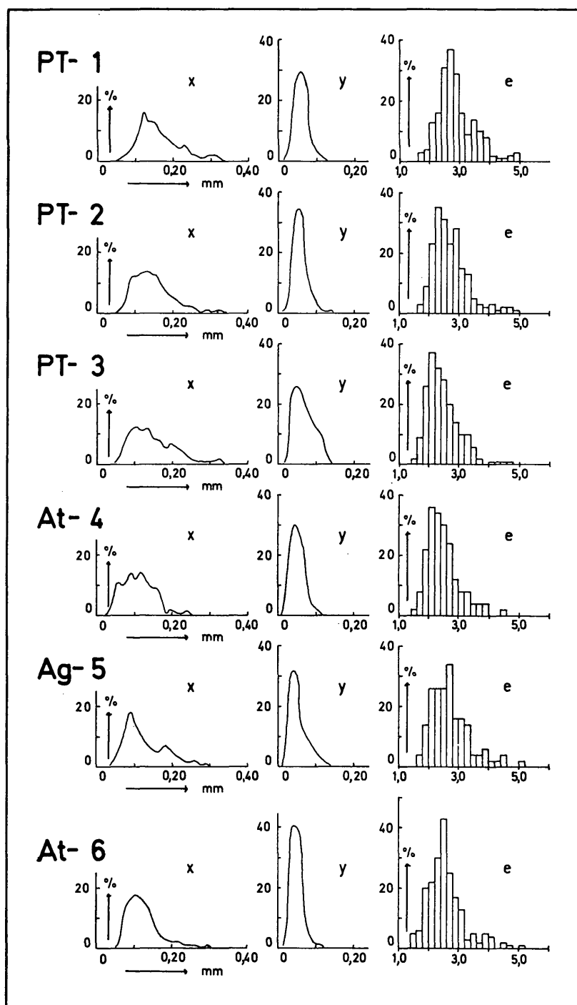
Abb. 3: Diese und die folgende Abb. 4 geben eine Übersicht über die Verteilung von Länge und Breite und Elongation der untersuchten Zirkone in den verschiedenen Gesteinen.
