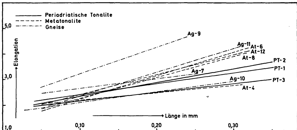
Abb. 2: Wachstumstendenz der Zirkone der untersuchten Gesteine.
