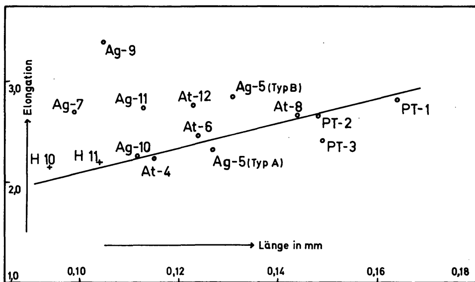
Abb. 5: Mittlere Länge im Vergleich zur durchschnittlichen Elongation der Zirkone der einzelnen Proben. Die Werte für die Proben H 10 (DK 10, Tonalit; Val Daone) und H 11 (DK 11, geschieferter Tonalit; Eingang ins Val Genova) sind der Arbeit von G. HOPPE 1962 entnommen.
