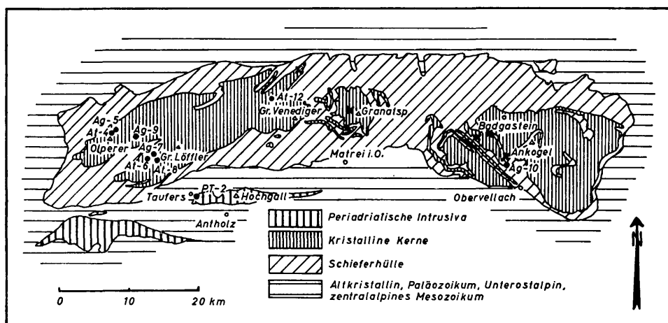
Abb. 1: Schematisierte geologische Übersichtsskizze der Hohen Tauern mit eingetragenen Probepunkten (Probe PT-1 und PT-3 liegen außerhalb des dargestellten Bereiches). Die Kreuzchen (×) geben jene Gesteine an, die vorwiegend metamiktische Zirkone zeigen, hier aber nicht näher behandelt werden.
