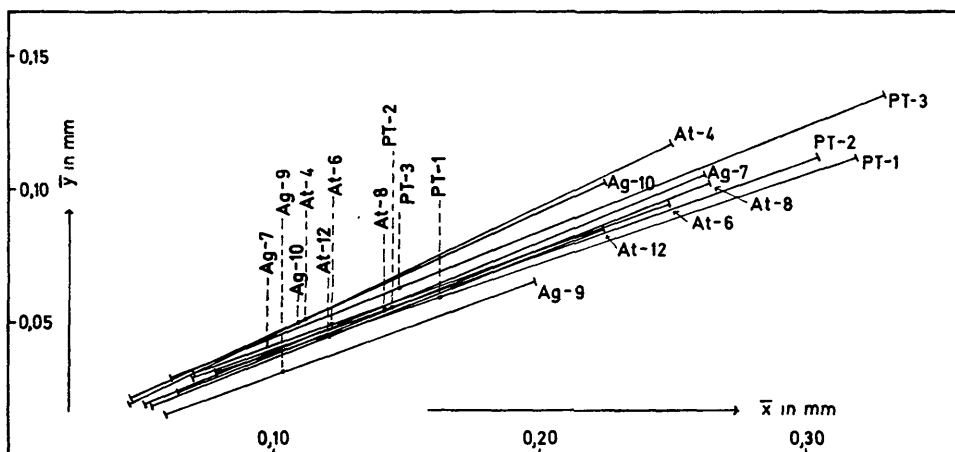
Abb. 6: RMA-Diagramm der bearbeiteten Zirkonproben.
