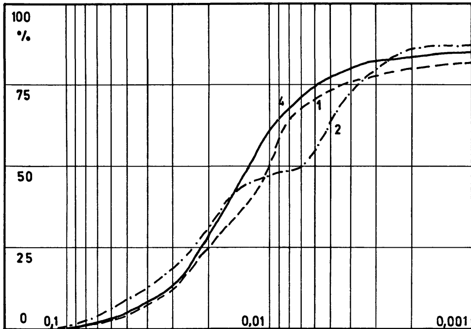
Abb. 6. Summenkurve der Lössse.
