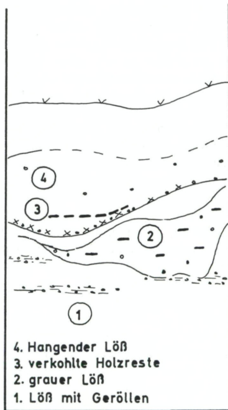
Abb. 5. Schematisches Profil durch die Grabung Ruppersthal (mit Angabe der Proben); Knochenlage (xx), Pflanzenreste (---) und Gerölleinstreuungen (ooo). Der obere Teil des Profiles ist mechanisch umgewälzt.
