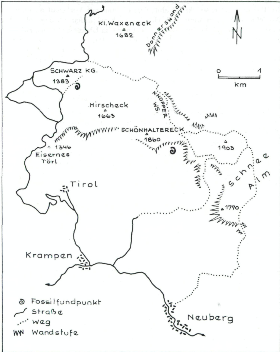
Abb. 1 Lageskizze mit Fossilfundpunkten. (nach LEIN in LEIN & ZAPFE, 1971).
