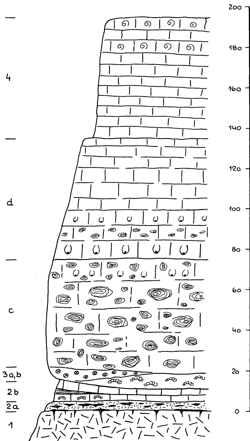
Abb. 2 Sammelprofil der Obertrias- Entwicklung des Schönhaltereck-Plateaus: 1 Wettersteindolomit, 2a Cidaris-Grenzdolomit, 2b Cidaris-Schichten, 3 „Dachsteinkalk“, 4 Hallstätterkalk. (nach LEIN in LEIN & ZAPFE, 1971).
