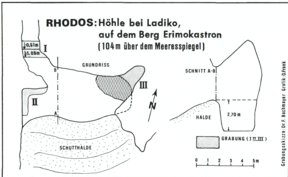
Abb. 2. Grund- und Aufriß der Höhle (Grabung I, II, III im Jahre 1973)
