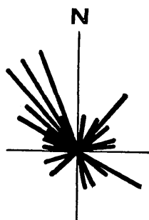
Abb. 3. Einregelung von Neomegalodon (N.) hoernesii ssp. (FRECH, 1904)
