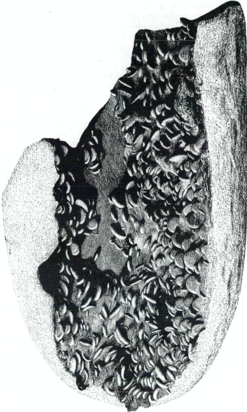
Abb. 2. Asthenopodichnium xylobiontum n. g. n. sp. Holotypus. Konkretion mit Lebensspuren (Spreitengänge) von Ephemeropterenlarven aus dem Jung-Miozän (Pannon E) von Hengersdorf bei Wien (NÖ.). Holzsubstanz zerstört, die im Holz angelegten Spreitengänge sind als Steinkerne erhalten. Original Naturhist. Museum Wien, Geol.-Paläont. Abt., Acqu. No. 1905/VII/8, ca. \frac{5}{6} nat. Größe
