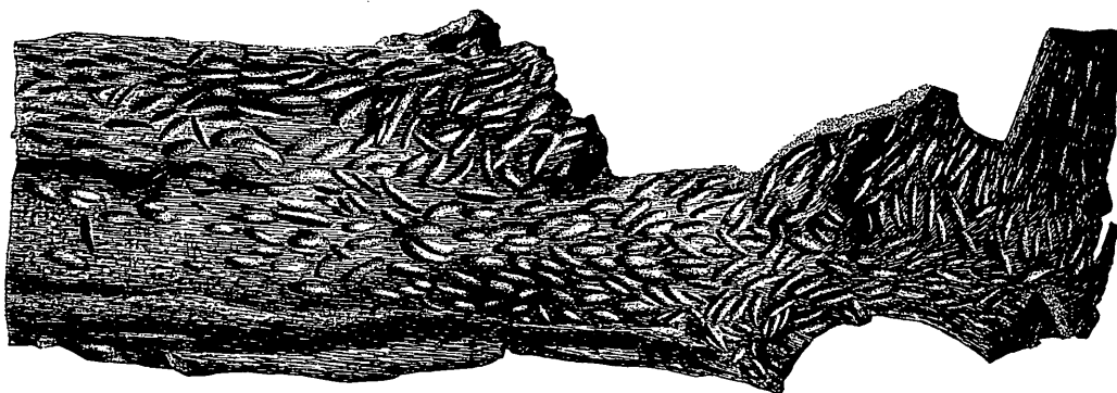
Abb. 1. Xylit aus dem Jung-Miozän (Pannon E) von Brunn—Vösendorf S Wien (NÖ.) mit den Lebensspuren von Ephemeroterenlarven ( Asthenopodichnium xylobiontum n. g. n. sp.). Beachte die Kerben an der Oberfläche des entindeten Holzrestes. Etwas verkleinert, Original Institut für Paläontologie, Universität Wien
