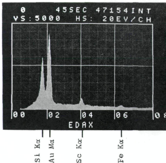
Abb. 1. Energiespektrum des goldbedampften Bazzits dieser Arbeit. Stereoscan Mark 2A (Cambridge Instruments) bei 20 KeV und mit EDAX 707
