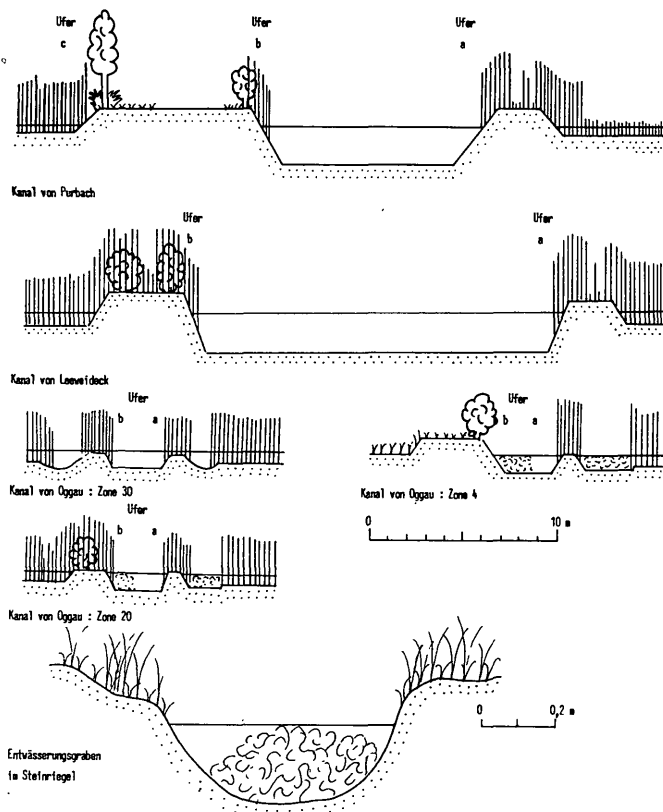
Abb. 2. Schematisierte Querschnitte der untersuchten Schilfkanäle (untereinander maßstäblich, Nordufer links) und eines Entwässerungsgrabens im Vorschilfwiesen-Bereich
