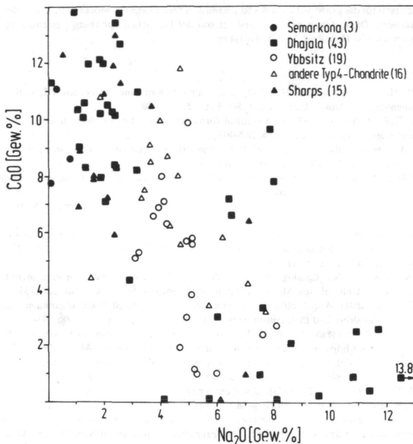
Abb. 2. CaO-Na 2 O-Variation von Al-reichen Chondren in Typ 3 und Typ 4 Chondriten. Chondren aus Typ 3 Chondriten sind durch ausgefüllte und Chondren aus Typ 4 Chondriten durch offene Symbole dargestellt. Bis auf sehr wenige Ausnahmen weisen Chondren aus Chondriten vom Typ 4 mittlere CaO- und Na 2 O-Gehalte auf, während die überwiegende Anzahl der Al-reichen Chondren von Typ 3 Chondriten entweder Na 2 O- oder CaO-reich ist. Die Anzahl der untersuchten Chondren ist in Klammern angegeben.
