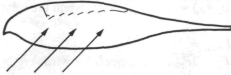
Abb. 3. Lage der freien Handschwingen im Abschlag und Anblasrichtung an der Flügelspitze, deren Orientierung durch das Verhältnis v/(\omega R) bestimmt ist
