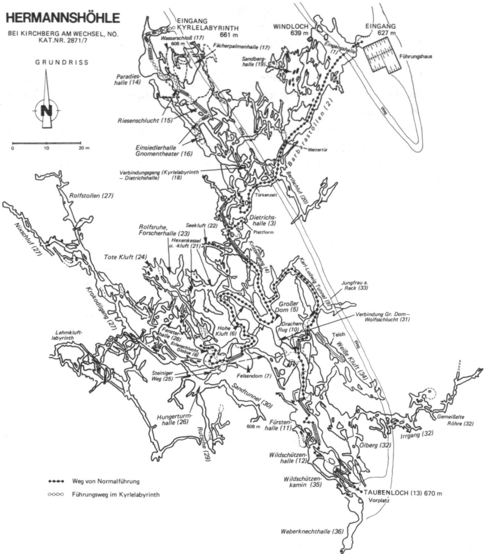
Abb. 1. Höhlenplan mit eingezeichneten Höhlenabschnitten und Führungswegen
