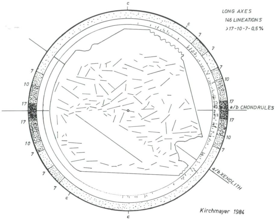
Abb. 7: Leoville-Chondrit der Photoaufnahme Tafel 1; 146 Lineationen = Längungen der Chondren und der Xenolithe sowie der kongruent deformierten Formelemente; ausgezählt > 17 — 10 — 7 — 0,5% des Durchmessers eines 1%-Auszahlkreises. Die gefügekundlichen b- und c-Koordinaten sind eingezeichnet, ebenso die ab-Ebene der Chondren und die davon verschieden liegende ab-Ebene des größten Xenolithen (Der kleinere Xenolith kann mangels Auflösungsvermögen nicht untersucht werden). Chondren-Tropie: 10%-Linie = 0,19.
