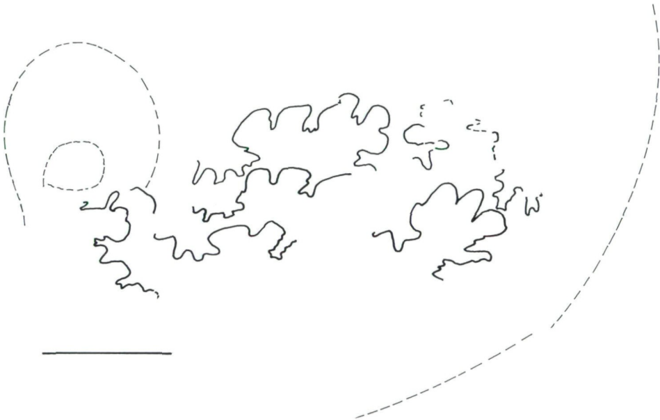
Abb. 9. Externsutura von Neptychites cephalotus (COURTILLER); NHMW 1992/83; Pichlbaueralm bei Unterlaussa, Oberösterreich, Fundstelle ULP 1 ; Maßstab = 10 mm.
