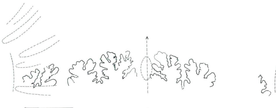
Abb. 10. Externsuture von Collignonicerias woollgari (MANTELL); NHMW 1989/52/36; Pichlbaueralm bei Unterlaussa, Oberösterreich, Fundstelle ULP 2 ; Maßstab = 10 mm.
