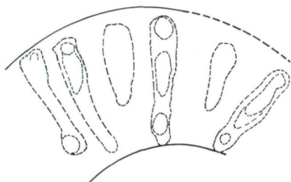
Abb. 5. Berippung von Kamerunoceras ganuzai (WIEDMANN); NHMW 1990/47/10; Pichlbaueralm bei Unterlaussa, Oberösterreich, Fundstelle ULP 1 ; Maßstab = 10 mm.
