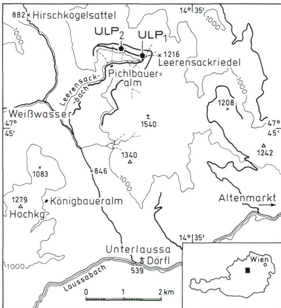
Abb. 1. Lageskizze der Fundstellen ULP 1 und ULP 2 .
