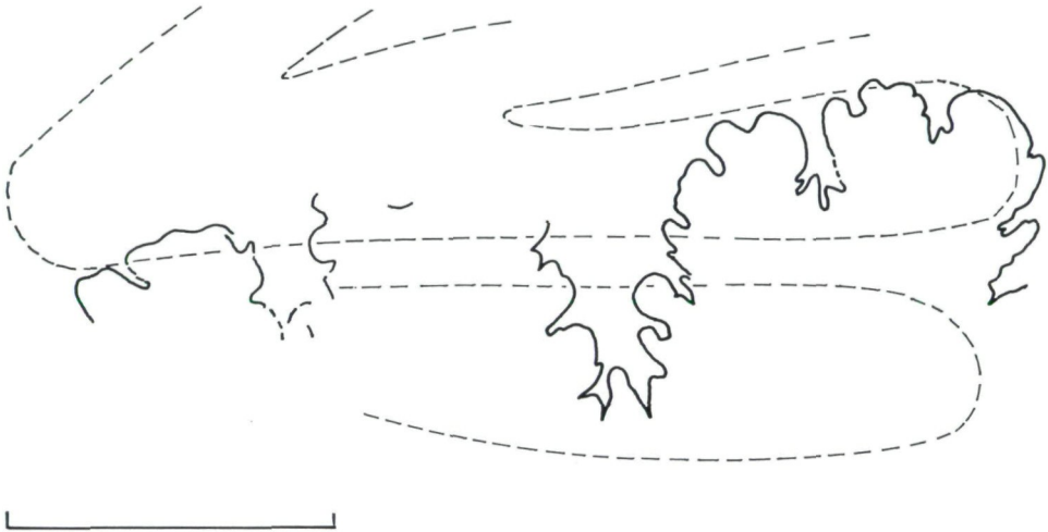
Abb. 8. Externsutura von Spathites (Jeanrogericeras) pachycostatus sp. nov.; NHMW 1989/27/6; Pichlbauralm bei Unterlaussa, Oberösterreich, Fundstelle ULP 1 ; Maßstab = 10 mm.
