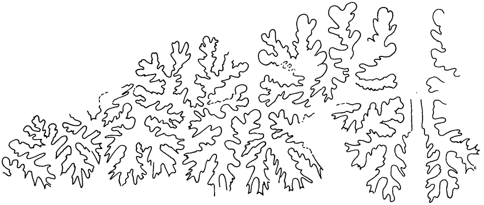
Abb. 4. Externsutura von Anagaudryceras cf. buddha (FORBES); NHMW 1990/47/8; Pichlbaueralm bei Unterlaussa, Oberösterreich, Fundstelle ULP 1 ; Maßstab = 10 mm.
