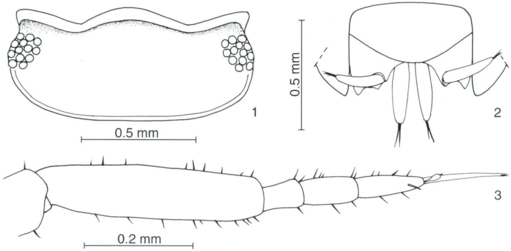
Abb. 1 - 3: Xeroporcellio pandazisi , ♂, 4,7 mm lang (aus SCHMALFUSS 1986). (1) Kopf von dorsal, (2) Telson und Uropoden, (3) distaler Teil der Antenne.
