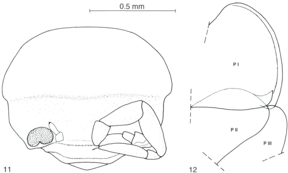
Abb. 11 - 12: Kithironiscus paragamiani gen.n., sp.n., ♀, Paratypus. (11) Kopf von dorsofrontal, rechte Antenne entfernt, (12) Pereion-Epimeren I - III des eingerollten Tieres.
