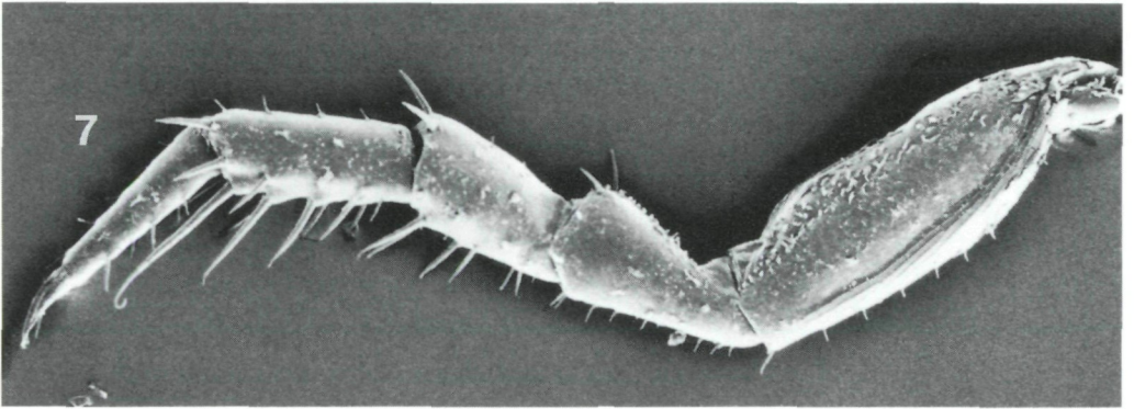
Abb. 6 - 7: Xeroporcellio pandazisi , ♂, Kefalliniá (SMNS T207). (6) Pereiopod I, Antennenputz-apparat an Carpus und Propodus, (7) Pereiopod VII.
