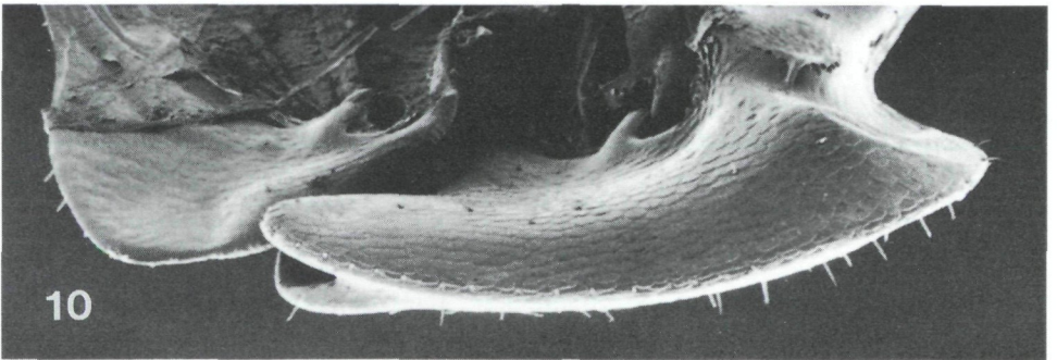
Abb. 8 - 10: Kithironiscus paragamiani gen.n., sp.n., Paratypen. (8) Eingerolltes Exemplar von lateral, (9) Pereion-Epimeren I und II von lateroventral, (10) Pereion-Epimeren I und II von medioventral.
