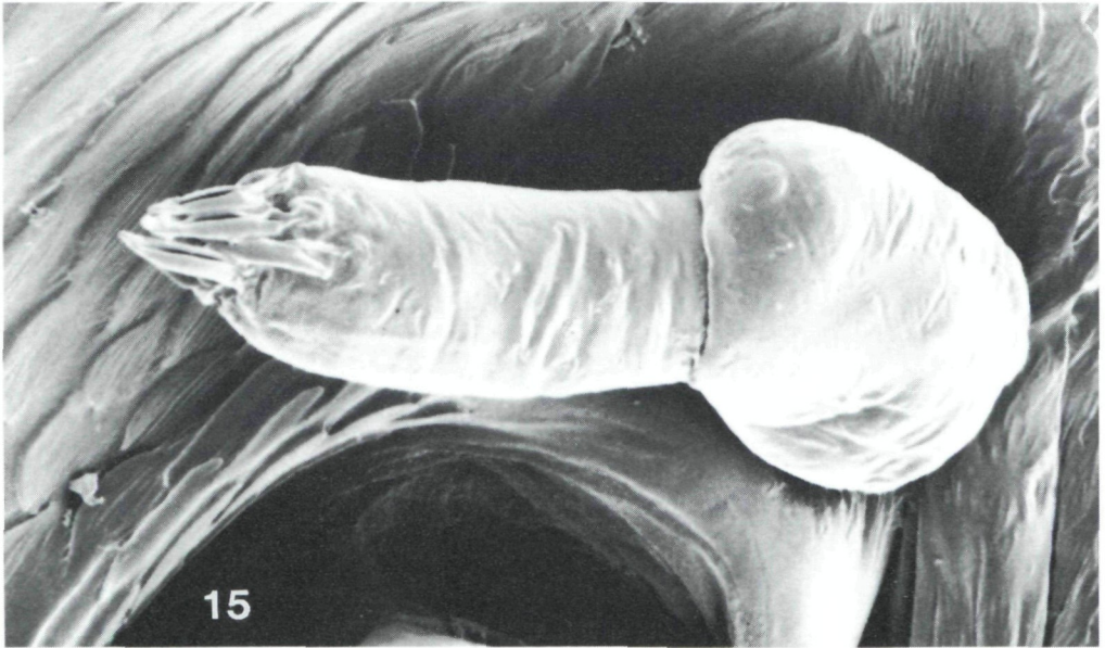
Abb. 14 - 15: Kithironiscus paragamiani gen.n., sp.n., ♀, Paratypus (14) Linke Antenne in situ, (15) Rechte Antennula in situ.
