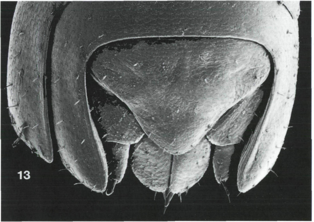
Abb. 13: Kithironiscus paragamiani gen.n., sp.n., Paratypus, Pleonotergit V, Telson und Uropoden in situ.
