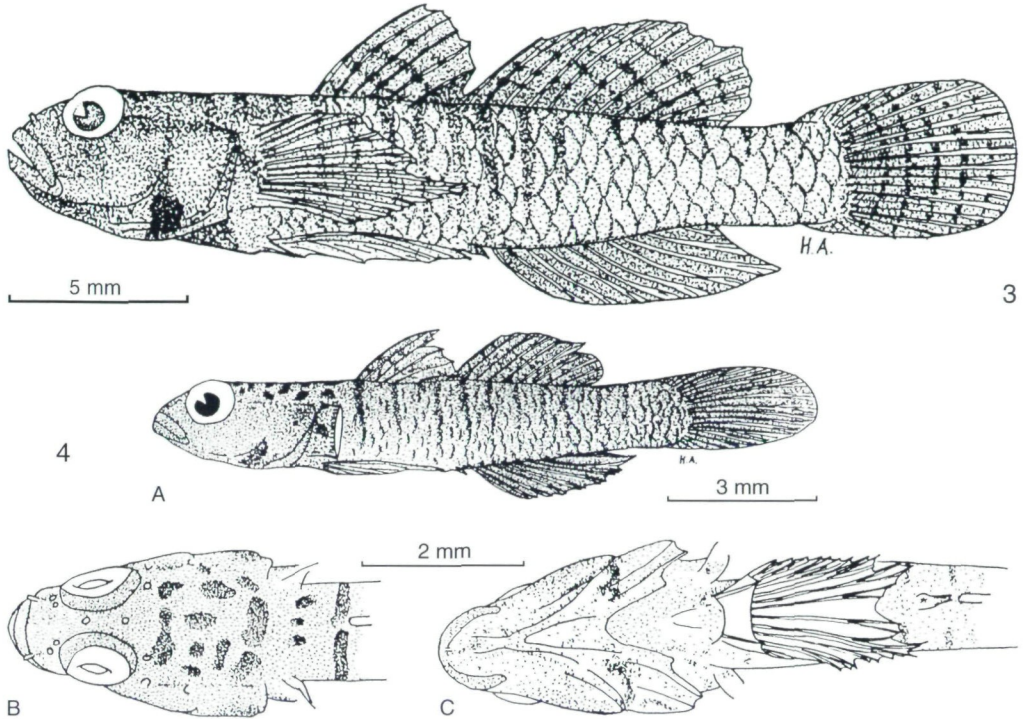
Abb. 3 - 4: Corcyrogobius liechtensteini , Männchen: (3) 24,0 + 5,5 mm. Ibiza, bei Portinatx; August 1991. (4) 17,1 + 4,9 mm. Ibiza, bei Portinatx; August 1991. A - Lateralansicht (Pectoralis nicht gezeichnet); B - Dorsalansicht des Kopfes; C - Ventralansicht.
