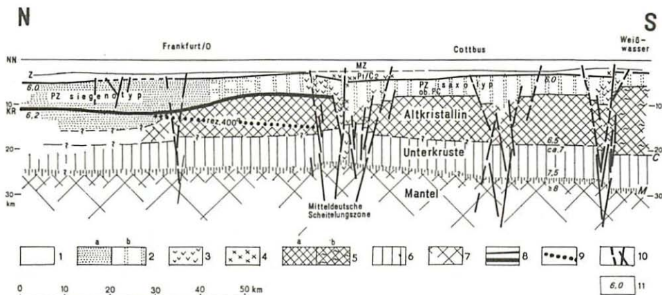
Fig. 4 Schematischer N-S-Schnitt.
