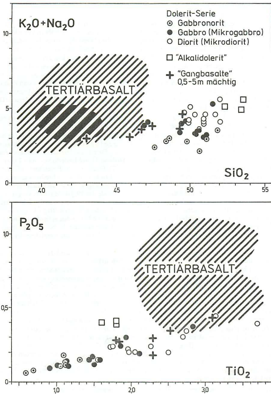
Fig. 1 Ausgewählte Parameter zur chemischen Klassifizierung der basischen Ganggesteinsformationen der Lausitz (Oxidgehalte in M.-%) Durch breite, aber kontinuierliche Schwankungen heben sich die Gesteine der Dolerit-Formation von den Tertiärvulkaniten (durchweg hohe Alkali- und TiO_2 -Werte) sowie von den „Alkalidoleriten“ mit wenig variierendem Gehaltswert ab. Unter den „Gangbasalten“ gibt es Vertreter, die sich bei den Doleriten und andere, die sich bei den Tertiärvulkaniten einordnen. Tertiärvulkanite nach PFEIFFER (1978), schematisiert.
