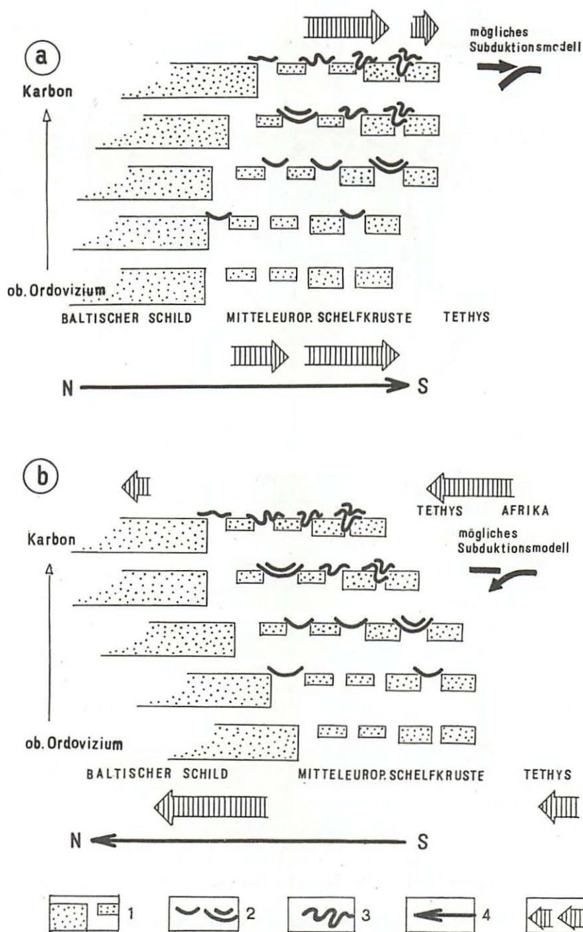
Fig. 3 Schema zur Frage der Driftrichtung im Paläozoikum Mitteleuropas.
