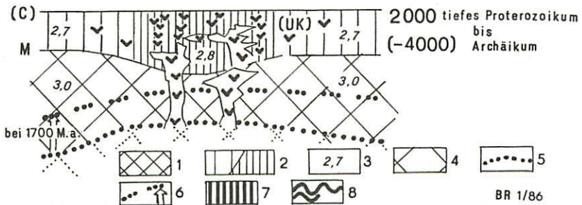
Fig. 6 Konzeptionsskizze zur Entwicklung des Vorpäälzoikums im Gebiet der Fig. 2. 1 Altkristallin der Oberkruste, 2 Unterkruste, rechts stärker basitbetont, 3 Durchschnittsdichte ( g/cm^3 ), 4 Oberer Erdmantel, im asthenosphärischen Bereich punktiert, 5 Grenze zur Asthenosphäre, Untergrenze der festen Lithosphäre, 6 Verschiebung dieser Grenze bei großräumiger Erwärmung, 7 Thermometamorphose, 8 Faltung, Tektonogenese
