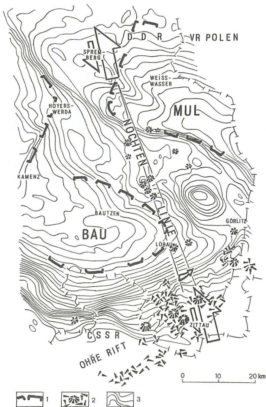
Fig. 8 Die Nochten-Linie als regionale Scherzone. 1 vorpaläozoische Teilblöcke: BAU Bautzener Teilblock, MUL Mulkwitzer Teilblock, 2 Neovulkanite, 3 vereinfachtes Schwerestrukturbild (ohne Maßangaben), Gradientzonen an alten Schollengrenzen und jungen Störungen
