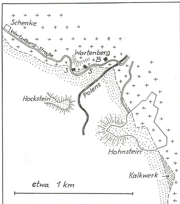
Fig. 2 Karte der Grenze von Granit (Kreuze) und Sandstein (Punkte) bei Hohnstein mit den Ansatzpunkten von COTTAS Schürfen (S) und Bohrung (B) an der Lausitzer Überschiebung bei Hohnstein (umgezeichnet nach COTTA 1838)
