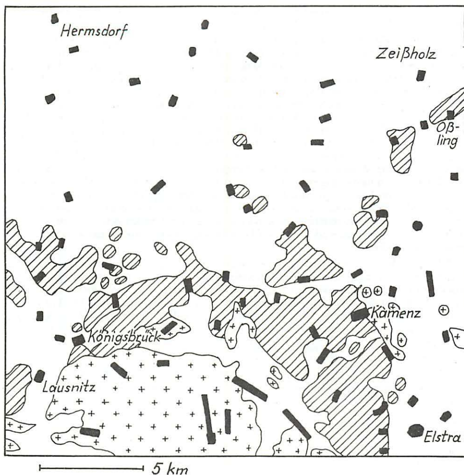
Fig. 4 Die Lage der Ortschaften (schwarz) im Raum Kamenz-Königsbrück in bezug auf die Verbreitung von Granit (Kreuze), Grauwacke (schraffiert) und Tertiär/Quartär (weiß). Umgezeichnet aus Sektion X (Dresden) der Geognostischen Spezialkarte des Königreichs Sachsen von C. F. NAUMANN und B. COTTA (1836-1845)
