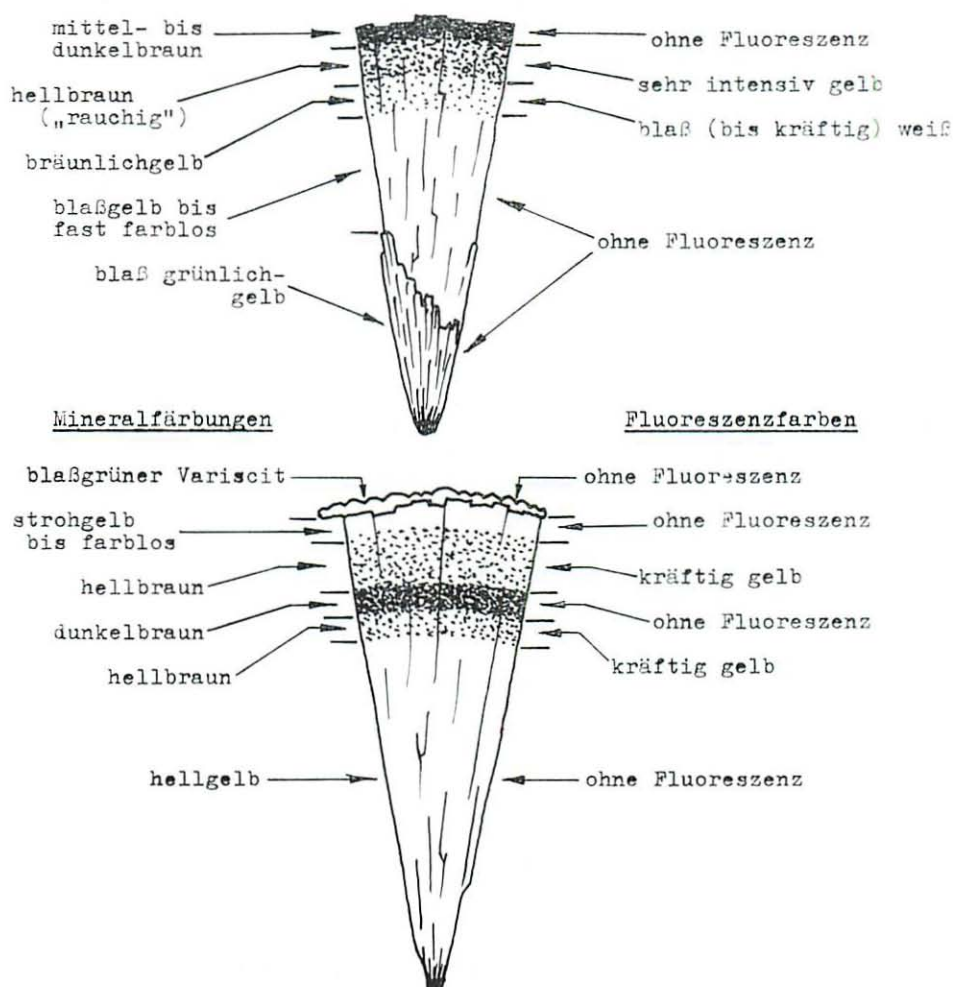
Abb. 5 Skizze zweier Wavellit-Kristallaggregate (Segmente aus kugeligen Wavellitaggregaten, Höhe 3 und 4 mm). Das untere der beiden Aggregate zeigt Reste einer Variscit-Überkrustung. Darstellung der Korrelation von Mineralfärbung (links) und Farbe/Farbintensität der Fluoreszenz bei Bestrahlung mit UV-Licht. Skizze: L. Nasdala
