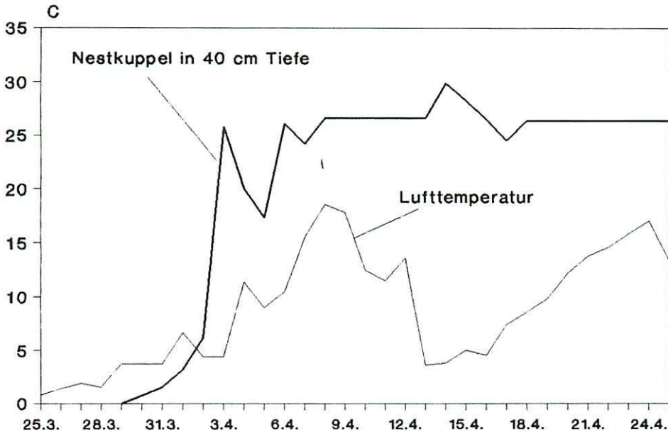
Abb. 3 Phänologie der Frühlingsaufheizung eines Nestes einer Waldameise aus dem Formica rufa/polyctena -Komplex im Frühjahr 1975 in der Gegend von Moskau (nach DLUSSKY 1980)
