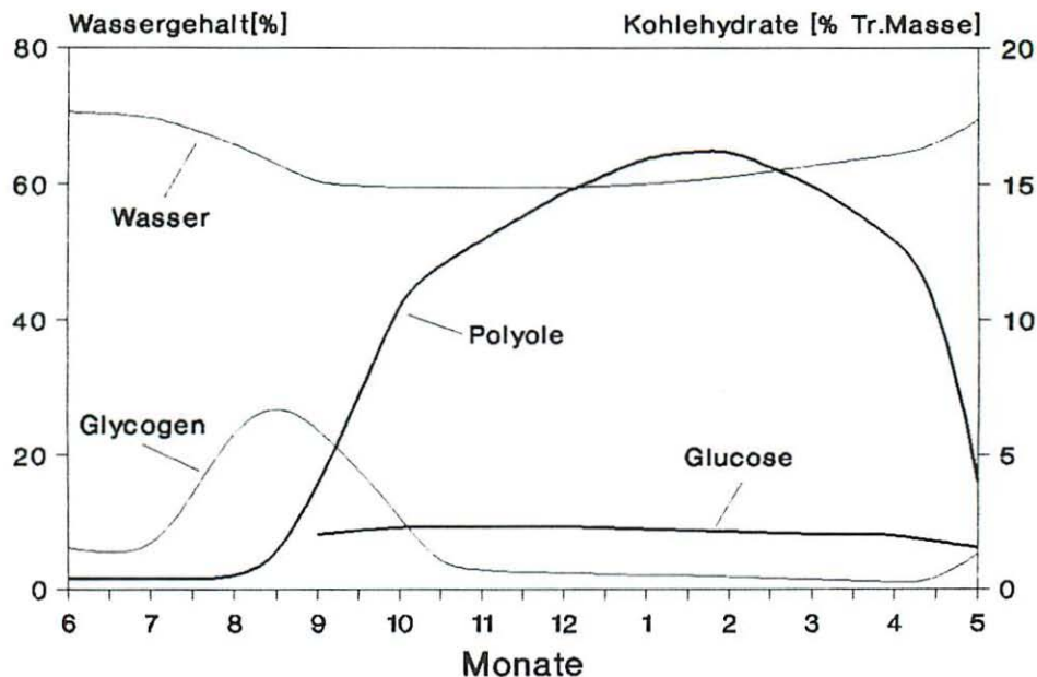
Abb. 2 Jahreszeitliche Veränderung des Wasser-, Glycogen-, Glucose- und Polyolgehaltes bei Arbeitern von Camponotus herculeanus (L.) aus dem Gebiet der Kolyma/Sibirien (nach BERMAN, SHIGULSKAJA & LEIRICH 1987, verändert). Der Wassergehalt ist in % der Frischmasse und die Kohlehydratgehalte in % der Trockenmasse ganzer Tiere angegeben.
