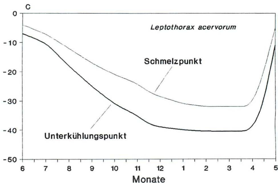
Abb. 1 Jahreszeitliche Veränderung des Unterkühlungs- und Schmelzpunktes bei Arbeitern von Leptothorax acervorum (Fabr.) aus dem Gebiet der Kolyma/Sibirien (nach BERMAN, SHIGULSKAJA & LEIRICH 1987, verändert)
