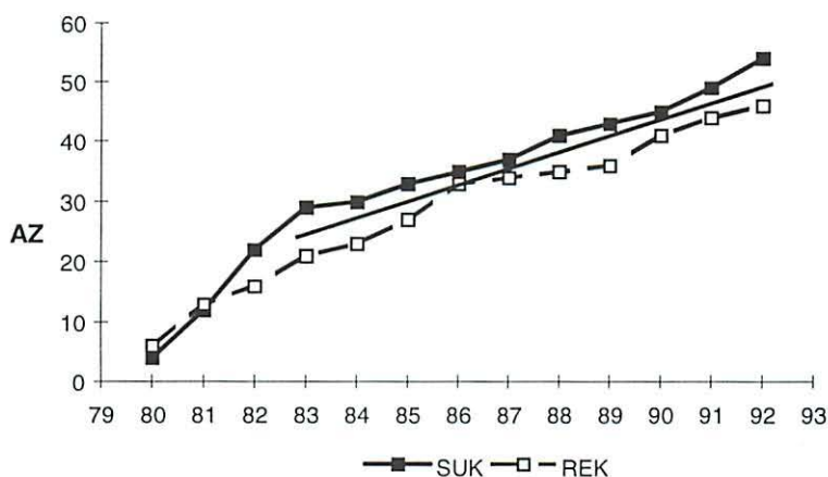
Abb. 2 Kumulative Artenzahlen der Gamasina-Taxozönosen auf SUK und REK. Die Regressionsgeraden von 1983 bis 1992 lauten: SUK: y = 27,4 + 2,7 \cdot x ( r^2 = 0,98 ), REK: y = 21,7 + 2,7 \cdot x ( r^2 = 0,97 ). AZ = Artenzahl (kumulativ), Zeitachse wie Abb. 1
