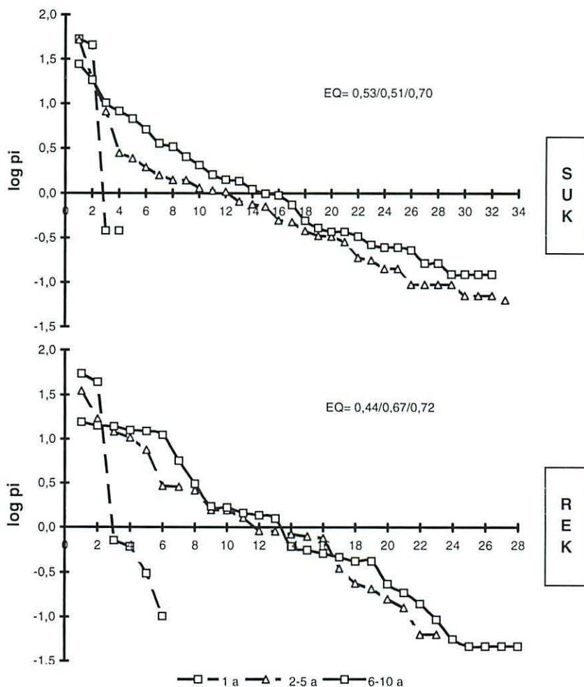
Abb. 3 Dominanzrangkurven der Gammasina-Taxozönosen von SUK und REK für 3 Sukzessionsabschnitte (1. Jahr, 2.-5. Jahr, 6.-10. Jahr); die jeweilige Äquität ( H'/H_{\max} ) ist angegeben. p_i = Dominanz in %
