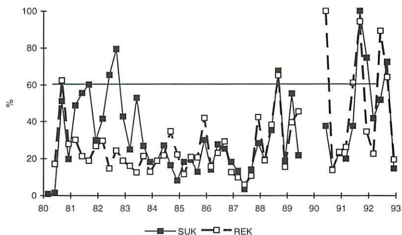
Abb. 1 Abundanzentwicklung der Gamasina auf den zwei Experimentalfächen SUK (ungestörte Sukzession) und REK (Rekultivierung durch Grasansaat und Mahd) in % der Maximalabundanz. Zeitachse 1980-1993
