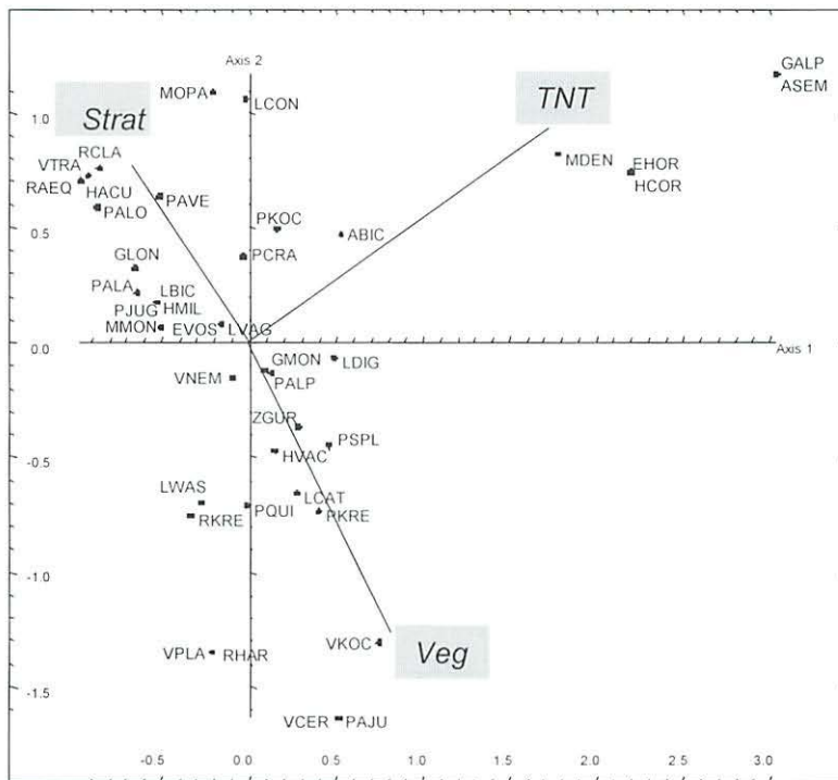
Abb. 1 Kanonische Korrespondenzanalyse der Gamasinen-Arten (Kürzel s. Tab. 1) unter Berücksichtigung von drei Umweltvariablen (TNT: TNT-Belastung des Bodens in \text{mg kg}^{-1} m.; Strat: Stratum; Veg: Vegetationstyp; vgl. 2)
