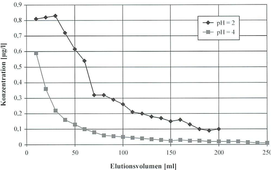
Abb. 1 Eluatkonzentration von Ni in Abhängigkeit vom Elutionsvolumen (Säulentechnik) (ZINKE 1996, ined.)
