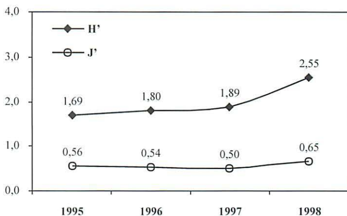
Abb. 3 Entwicklung der Diversität (Shannon-Index- H' ) und der Evenness ( J' ) der Gamasina-Synusie auf der Sukzessionsfläche S-I in den aufeinanderfolgenden Untersuchungsjahren von 1995 bis 1998
