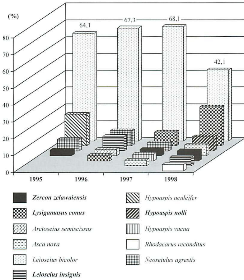
Abb. 2 Dominanzstruktur der Gamasina Arten nur mit D > 3,2\% auf der Sukzessionsfläche S-1 in den Jahren 1995 bis 1998. Die Gamasina-Waldarten sind fett markiert
