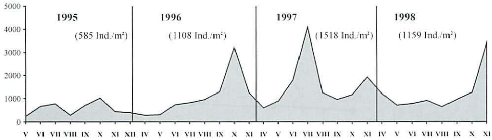
Abb. 1 Abundanzentwicklung der Gamasina (Ind./m²) auf der Sukzessionsfläche S-1 in den Jahren 1995 bis 1998. Die mittleren Jahresabundanzen sind in Klammern angegeben
