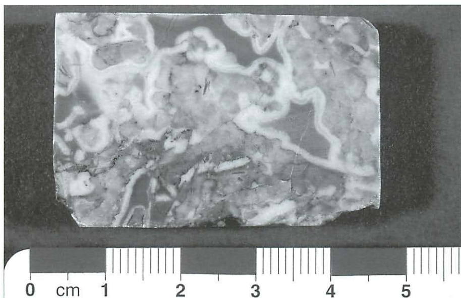
Abb. 25 Rotbraune Hohlraumfüllungen (dunkelgrau) mit weißen Kalzitziementsaum in Riffschuttalk (hellgrau) der Bol'soj Thač-Kalk-Folge. Anschliff der Probe 97/18 (Inv.-Nr. 10568c). Plateauoberseite des Bol'soj Thač, kleine Klippen 1 km SW der Knâžeskaâ-Wiese bei ca. 1950 m (Foto: O. Tietz).
