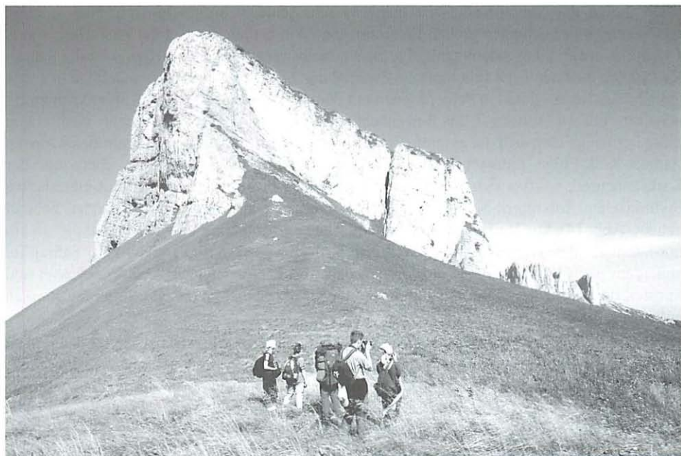
Abb. 12 Schichtstufe der Malyj Thač-Kalk-Folge. SE-Pfeiler des Malyj Thač Berges. Deutlich ist das Einfallen der Kalkfolge nach rechts (Nordost) zu sehen, im Hintergrund tauchen die Spitzen des Bol'soj Thač Berges mit seinem Gipfel auf (Foto: O. Tietz) s. a. App. 2, Fig. A2-6.
