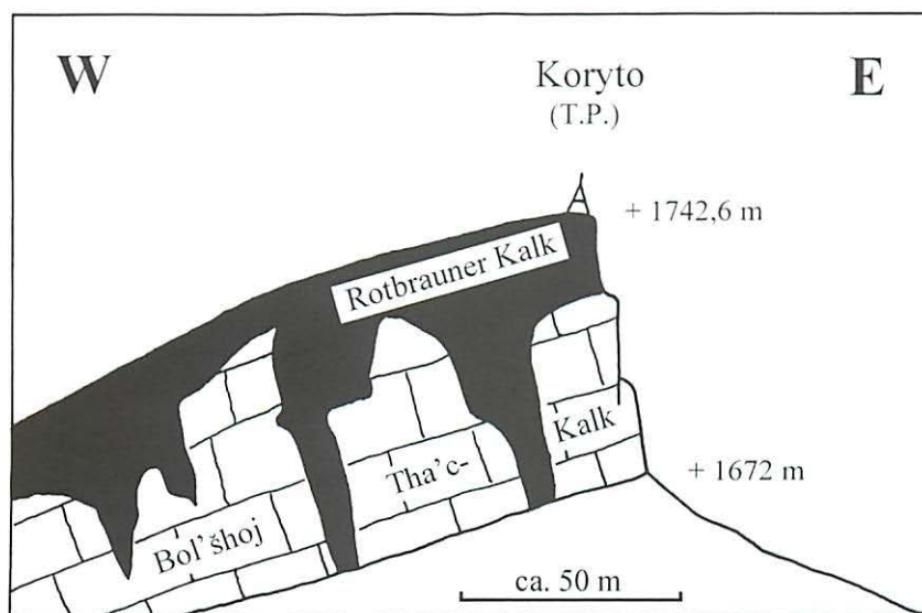
Abb. 30 Schematische Darstellung der Verbandsverhältnisse der beiden oberen triassischen Kalk-Folgen am Koryto-Berg, 7 km NW des Bol'soj Thač-Gipfels (Dokumentation vom 2.7.1997)
