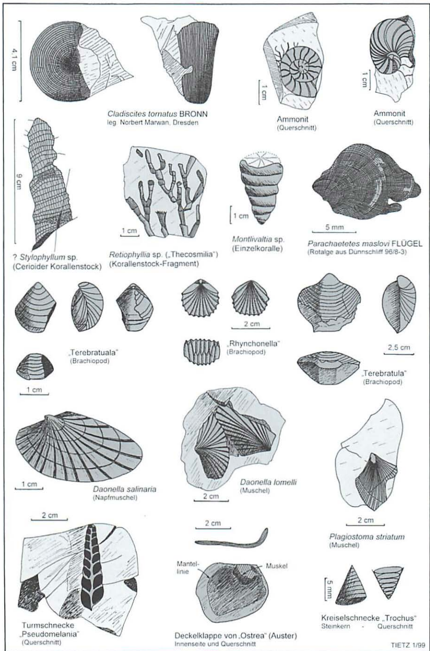
Abb. 20 Makrofauna der Bol'soj Thaç-Kalk-Folge (Norium-Stufe), zusammengestellt aus Lese- steinen der Schotterfelder unterhalb der Südwestflanke des Bol'soj Thaç Plateaus
