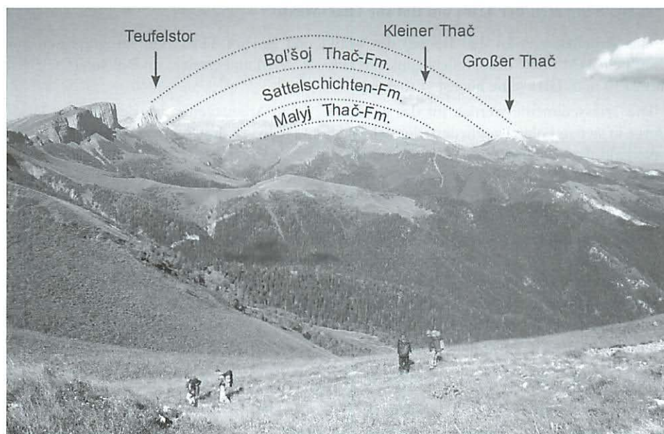
Abb. 6 Blick in die aufgebrochene Antiklinalstruktur des Triasvorkommens im NW-Kaukasus. Aufnahme vom Sunduki-Berg nach Nordwesten (Foto: O. Tietz) s. a. App. 2, Fig. A2-3.
