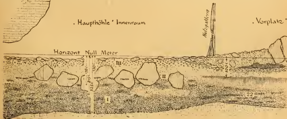
Längsprofil durch die Haupthöhle (im Grundriß „Profil a“).
