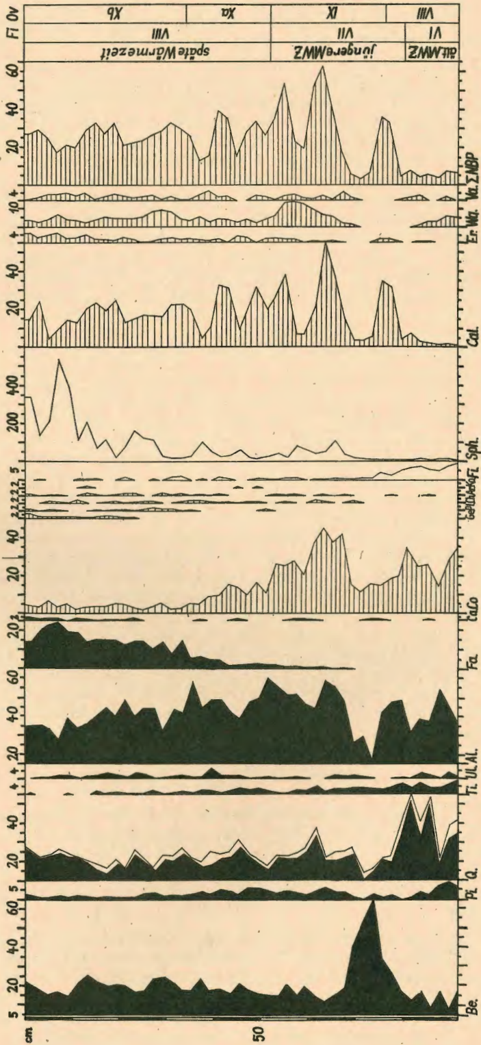
Abb. 4: Pollendiagramm des Torfprofils II. Aus Platzgründen sind in folgenden Kurven Bereiche der Kurvenflächen weggelassen:
