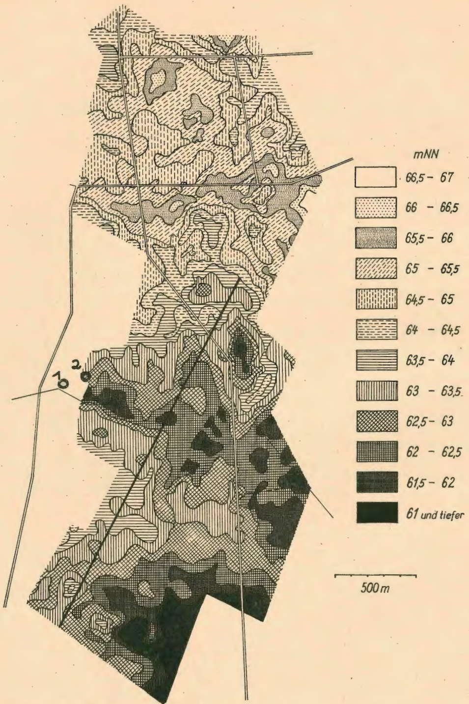
Abb. 1: Relief des Mooruntergrundes (nach Unterlagen des Torfwerkes Klasmann). Die Punkte 1 und 2 im Westteil bezeichnen die Entnahmestellen der beiden hier beschriebenen Torfsäulen. Die von Südwest nach Nordost verlaufende starke Linie entspricht der Lage des in Abb. 2 wiedergegebenen Profilschnittes.
