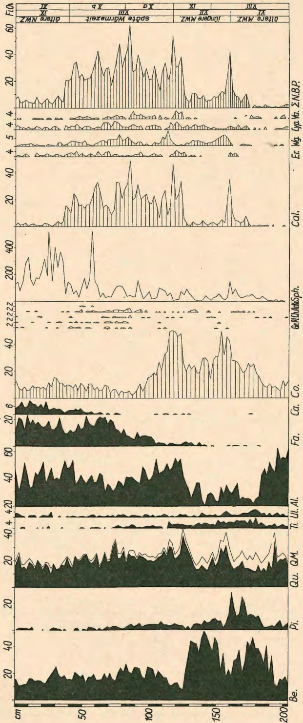
Abb. 3: Pollendiagramm des Torfprofils I.
