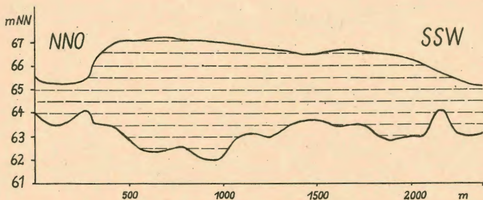
Abb. 2: Profilschnitt durch das Weiße Venn (Zustand 1924, nach Unterlagen des Torfwerkes Klasmann) längs der in Abb. 1 markierten Linie.
