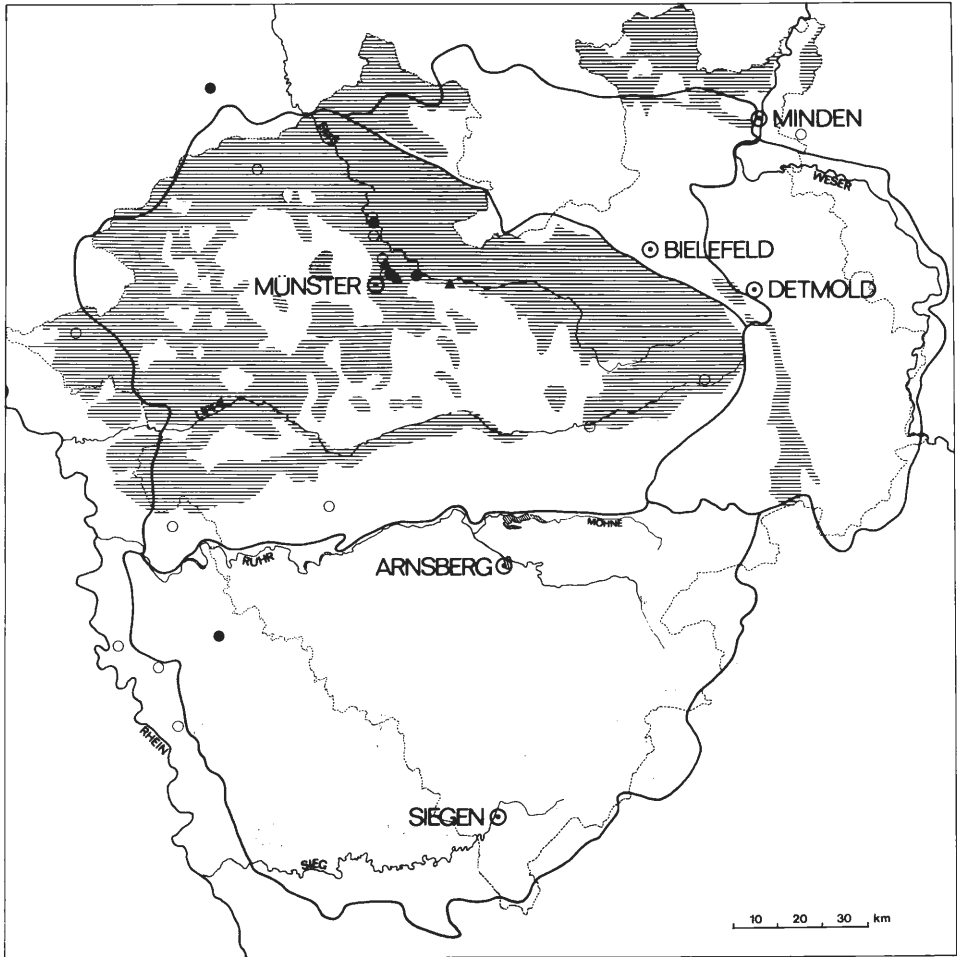
Abb. 2: Hypocaccus rugiceps . Symbole wie in Abb. 1. Die schraffierten Gebiete stellen Sand- und Niedermoorböden dar.
